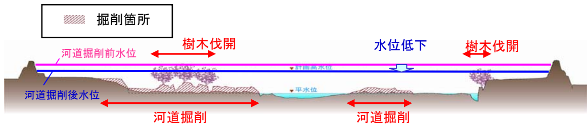
河道掘削のイメージ
