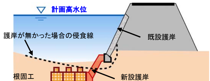
急流対策のイメージ
