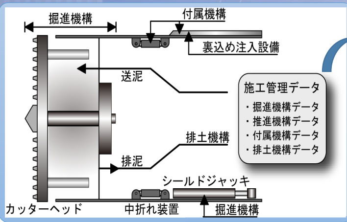
シールドシステム概要(泥水式)
