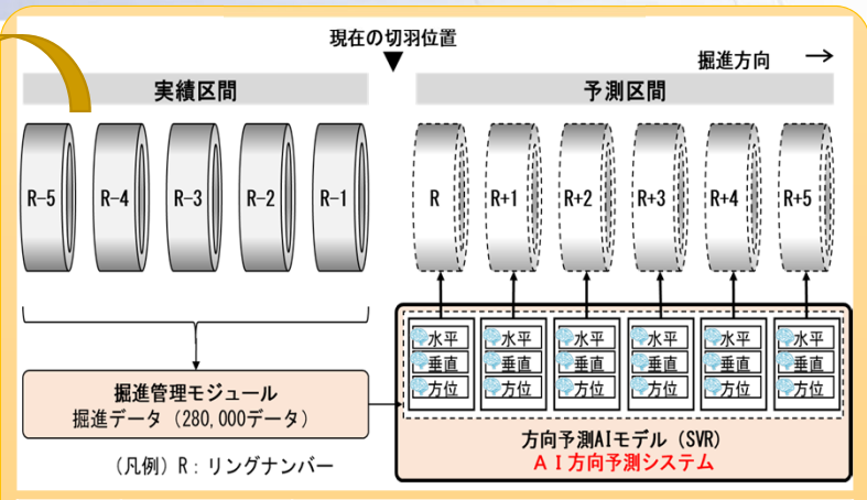
方向予測AIモデル
