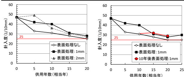
図-1 促進耐候性試験での針入度変化
