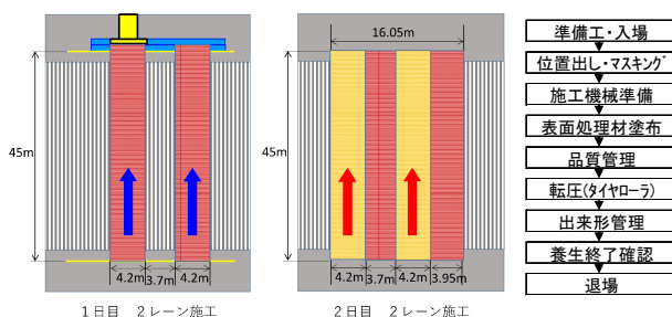
図-4 施工平面図と施工フロー
