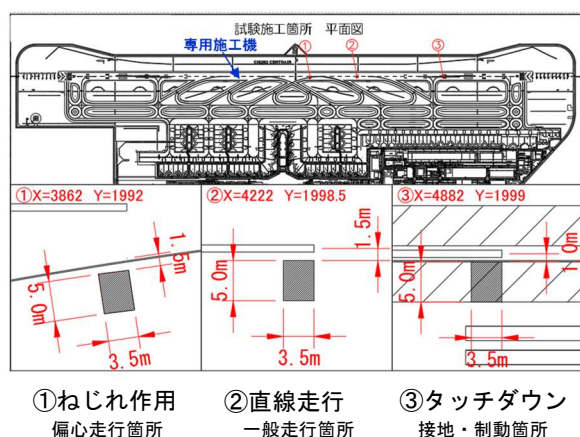
図-2 滑走路試験施工位置
