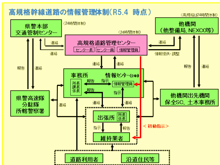
図-2 高規格道路管理センターの情報連絡体制
