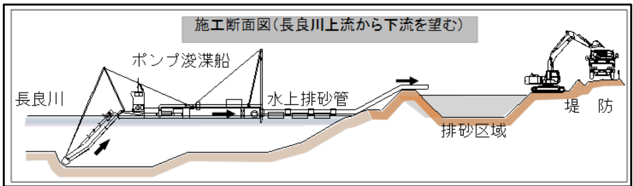
図-2 しゅんせつ工事の作業イメージ
