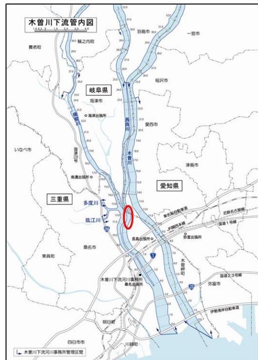
図－１ しゅんせつ工事位置図
