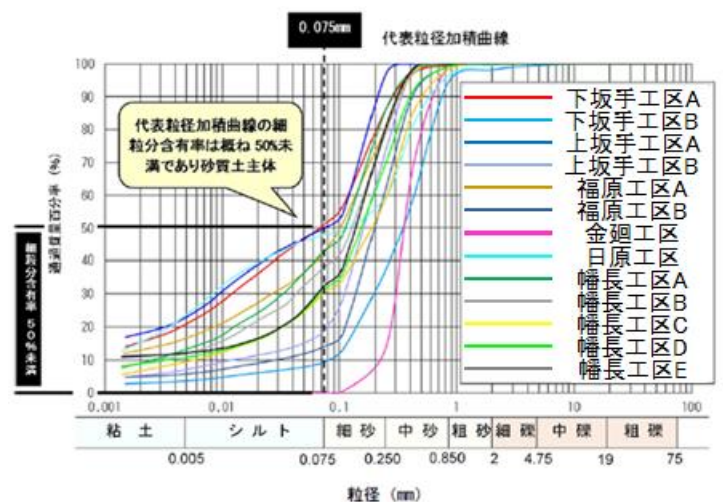
図-3 代表粒径加積曲線集積図
