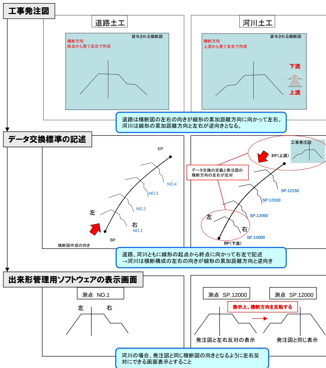
図-2 舗装工（河川）の横断形状の向き
