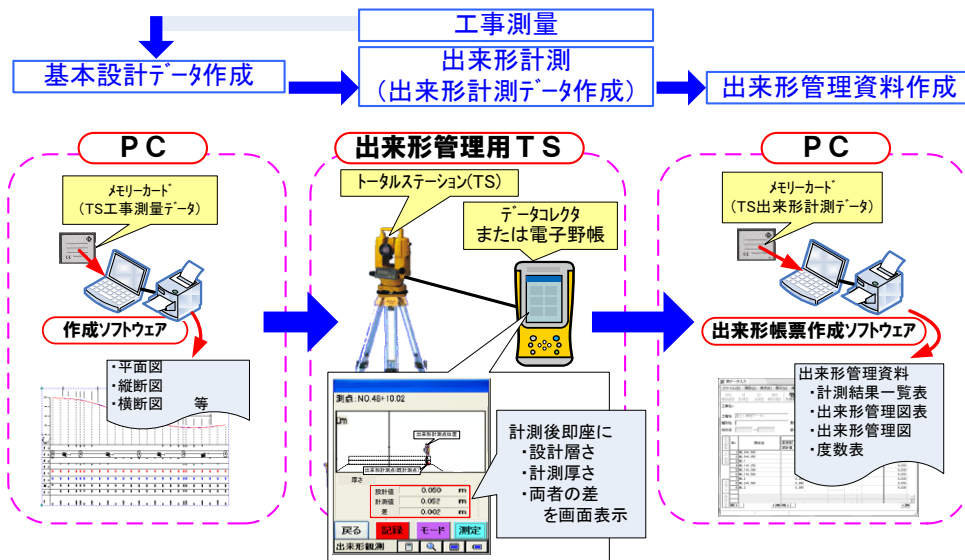
図-1 機器の基本構成 (例)
