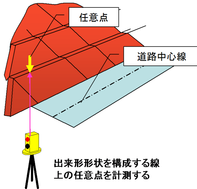
図-6 任意断面での出来形確認イメージ
