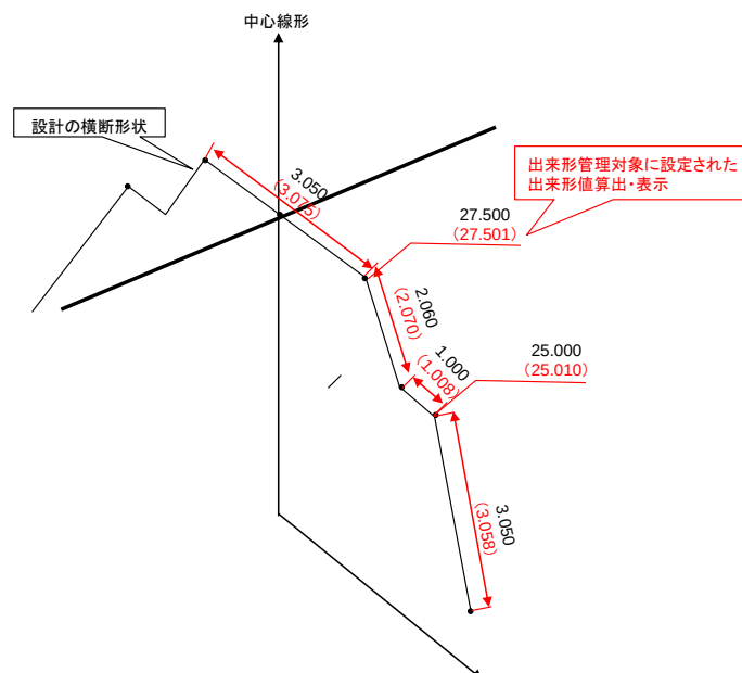
図-12 横断図作成方法（出来形計測結果を含む）
