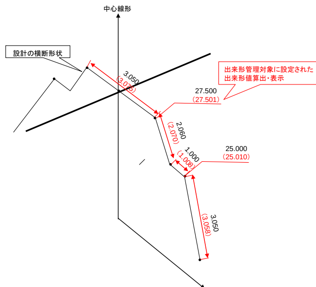
図-156 横断図作成方法（出来形計測結果を含む）
