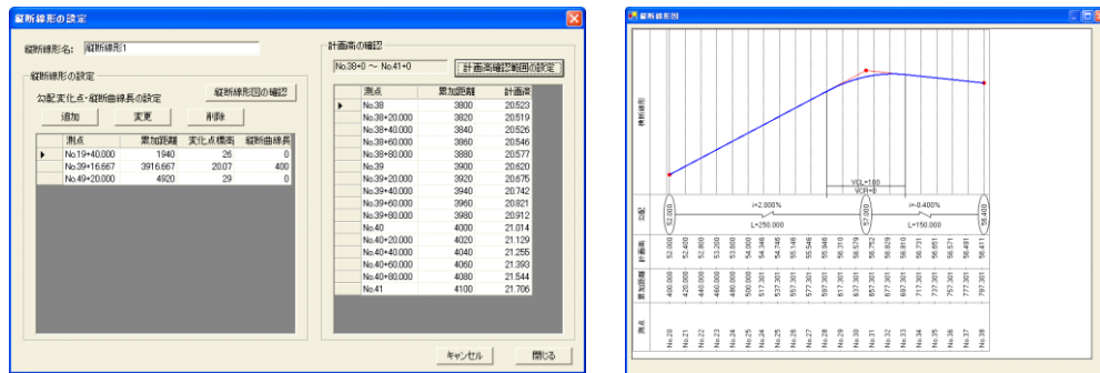
図-6 縦断面データの入力・確認と縦断面図確認画面例
