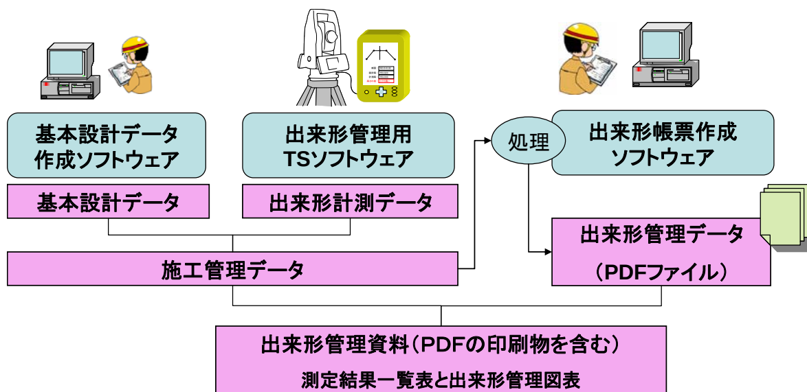
図ー 2 出来形管理用T Sにおけるデータの流れ
