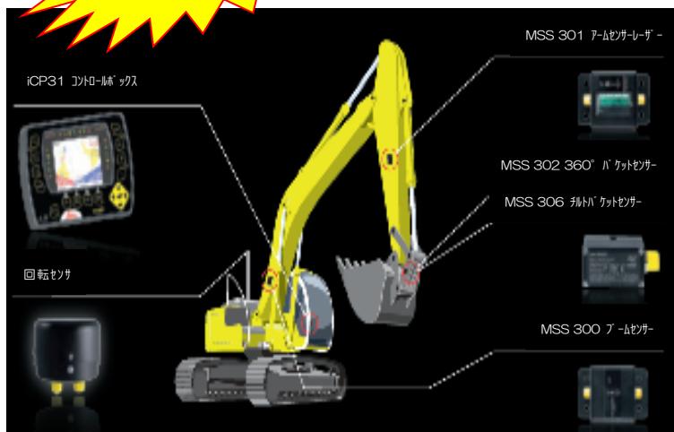
☆2D マシガタシステムバックホー
