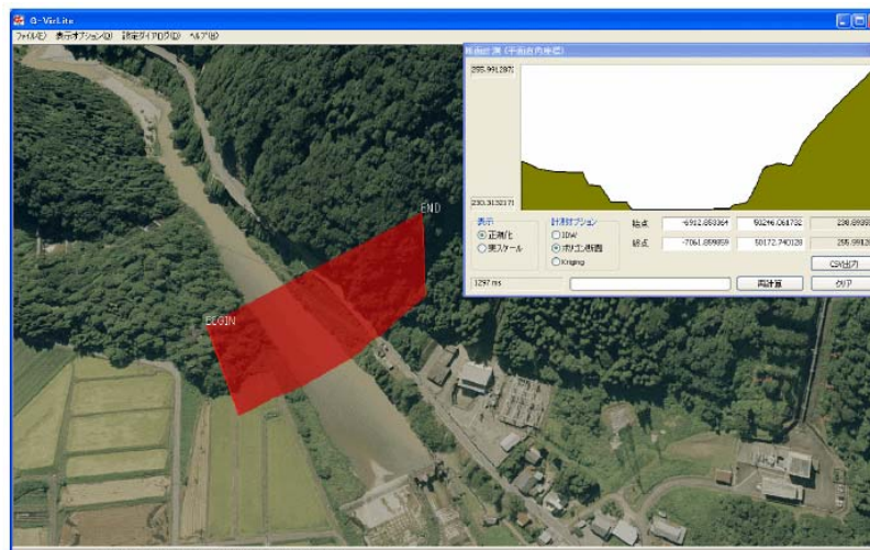
【3次元空間計測・情報管理システムでの表示例（データ提供：国土交通省近畿地方整備局九頭竜川ダム統合管理事務所）】
