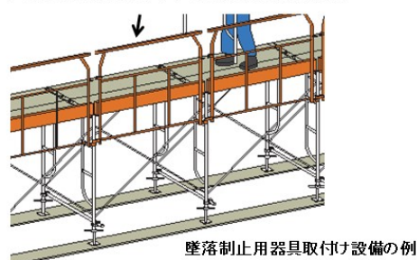
手すり先行工法による手すりわく(優先的に指導)
