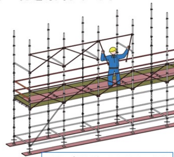
くさび緊結式足場の例
