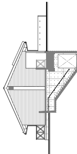
東 立面図 S=1:100
