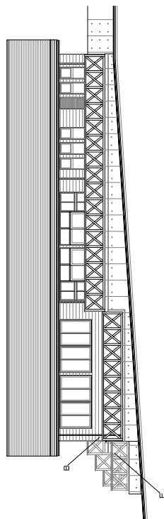
南 立面図 S=1:100
