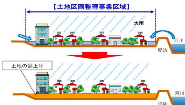
図 面的な土地の嵩上げのイメージ (出典：国土交通省「水災害リスクを踏まえた防災まちづくりのガイドライン」令和3年5月)
