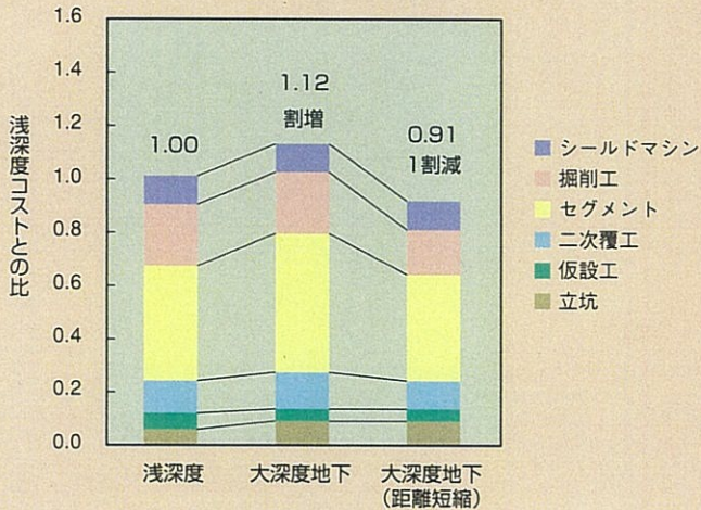
●大深度地下利用に当たっての建設コスト試算 (トンネル径10m、延長5,000mの場合/距離短縮25%)
