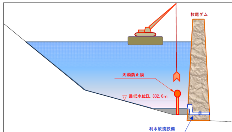
汚濁防止膜設置イメージ図
