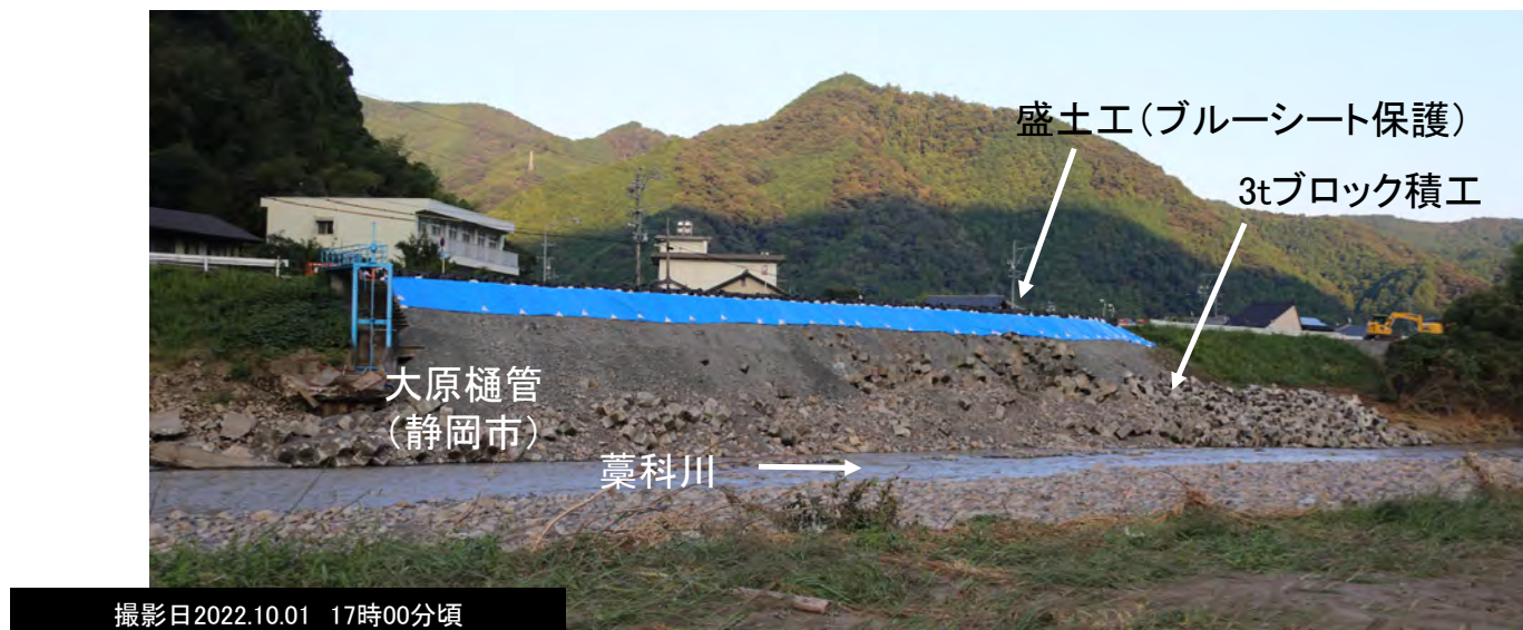
応急復旧後の状況
