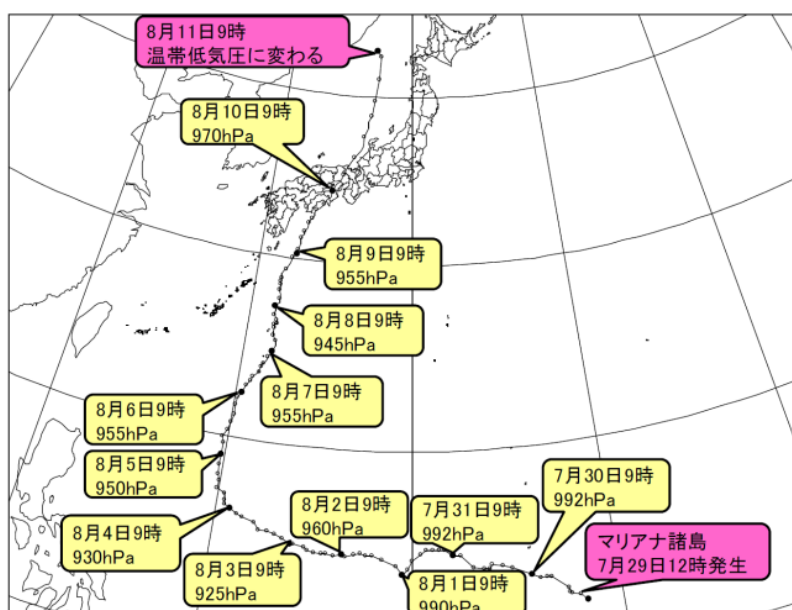
台風経路図
