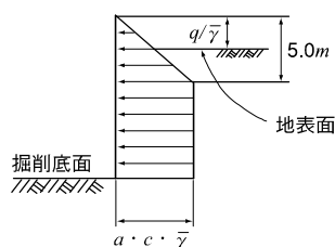
(b) 粘性土地盤土圧
