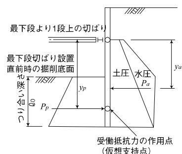
(b) 最下段切梁設置直前の計算
