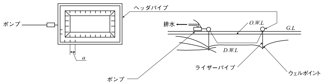
図 1-3-4 ウェルポイント工法
