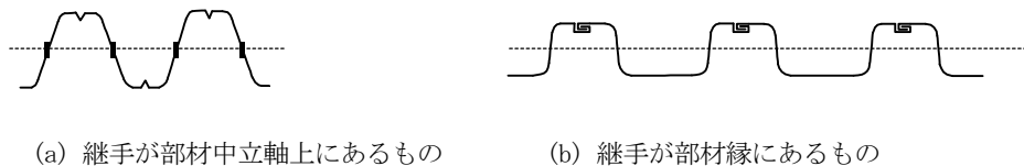
図 1-2-45 軽量鋼矢板継手位置図
