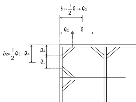
図 1-2-57 軸力を考慮する腹起しの軸力分担幅
