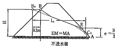
図 1-3-10 堤体の浸透モデル
