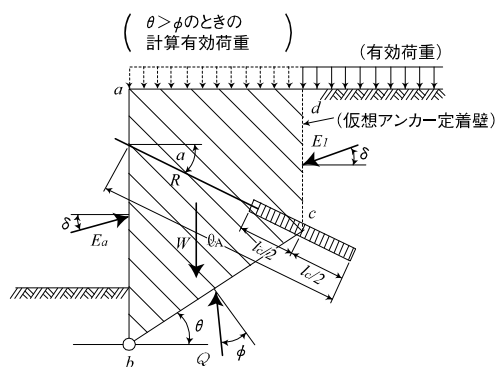
(山留め壁の仮想支持点)
