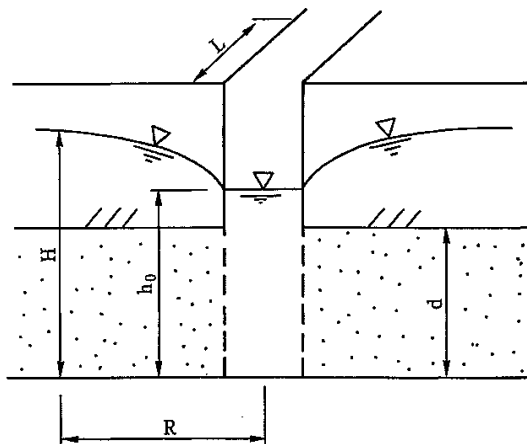
図 1-3-26 被圧帯水層（完全貫入状態）の概念図
