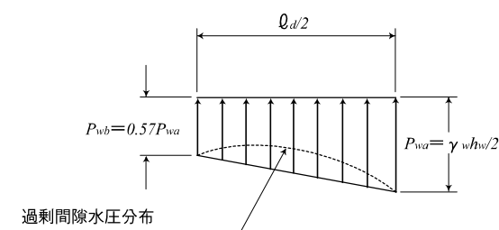
図 1-2-73 過剰間隙水圧分布
