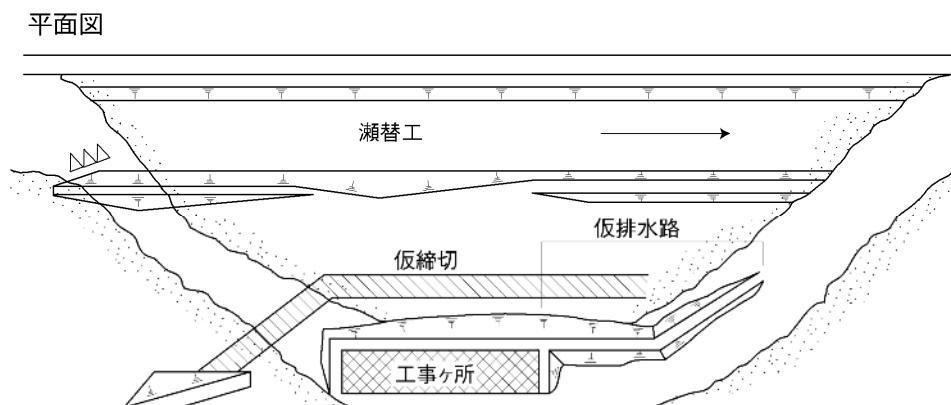
図 1-2-16 対策工例（仮排水路）
