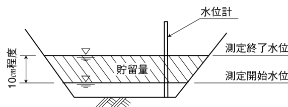
図 1-3-29 回復法による測定
