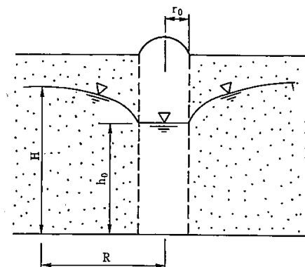
図 1-3-17 不圧帯水層（完全貫入状態）の概念図
