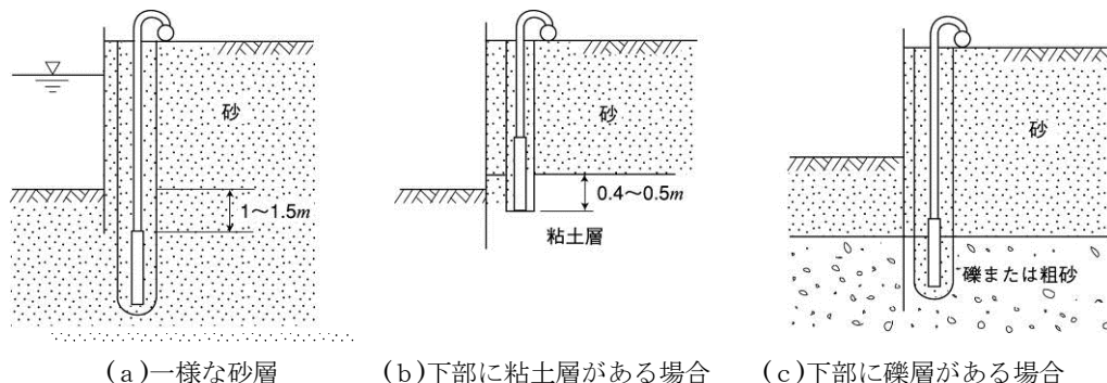
図 1-3-37 ウェルポイントの設置例
