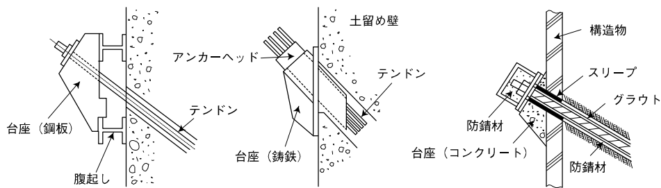
図 1-2-86 アンカー頭部形状の一例 [アンカー設計基準 6.4]
