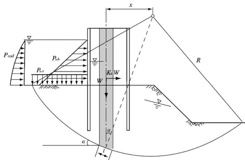
図 1-2-39 円弧すべり検討モデル
