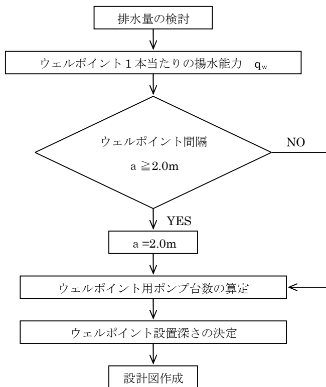
図 1-3-35 設計手順
