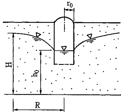
図 1-3-19 不圧帯水層（不完全貫入状態、井底からのみ排水）の概念図
