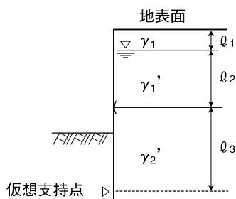
図 1-2-7 土の平均単位体積重量の求め方
