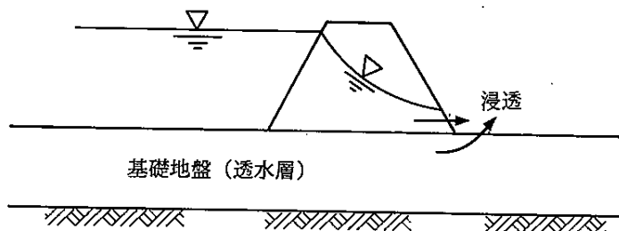
図1-3-9 堤体の浸透モデル概念図
