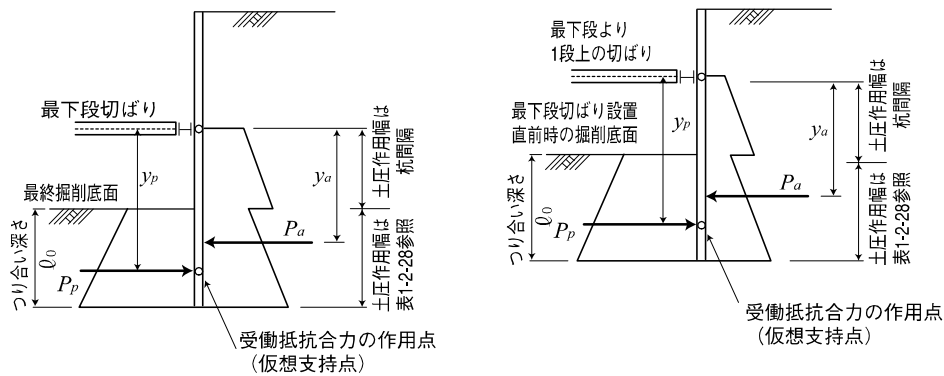
(a) 掘削完了時の計算 (最下段切梁位置での計算)
