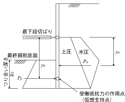
(a) 掘削完了時の計算
