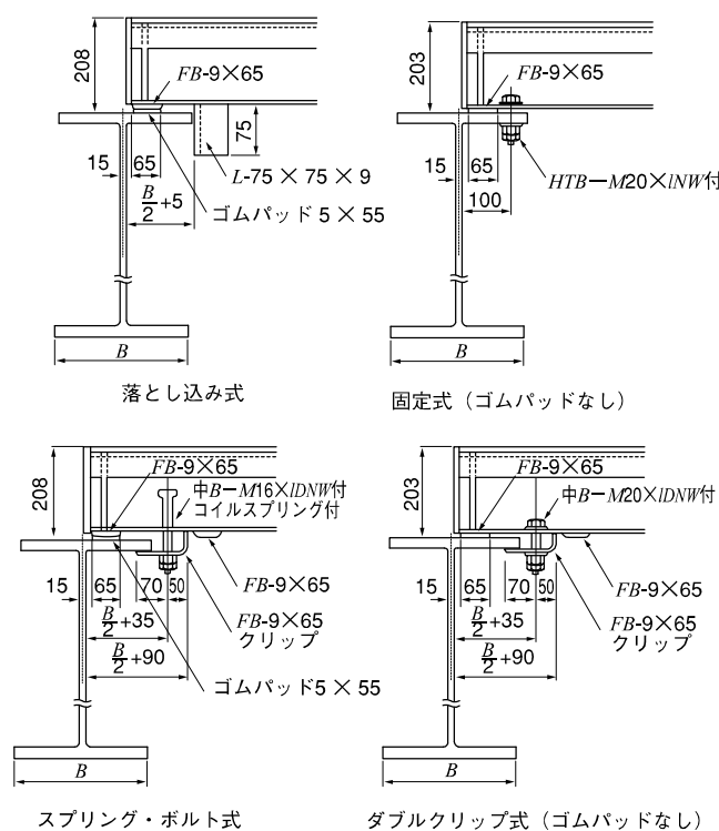
図 1-5-9 鋼製覆工板の設置例
