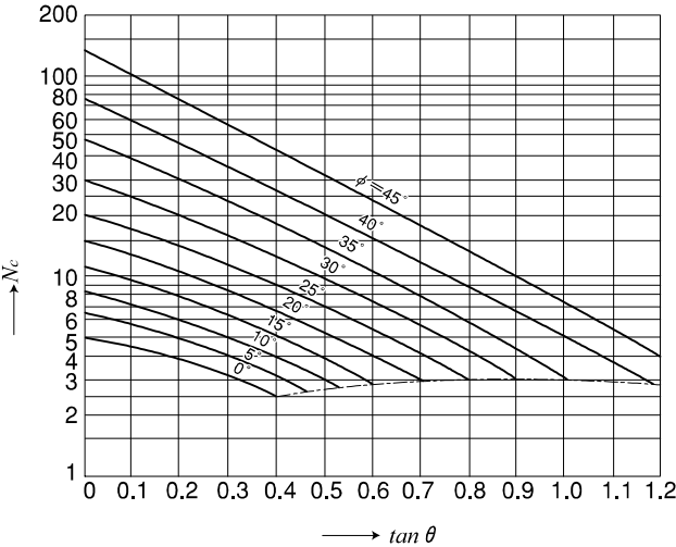
図 1-2-37 支持力係数 N_c を求めるグラフ
