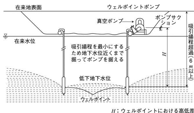
図 1-3-36 ウェルポイントの有効な設置位置
