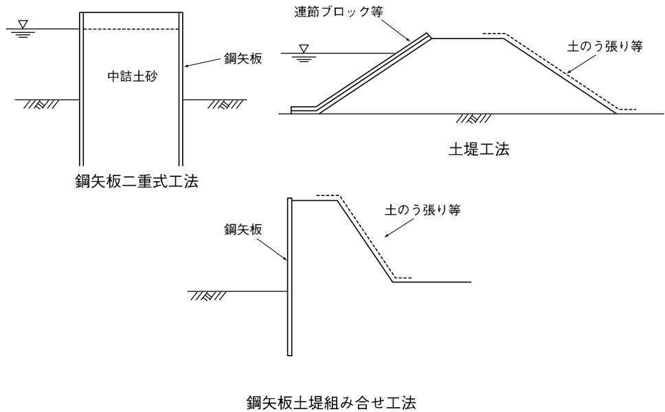
図 1-2-15 仮締切工法（例）
