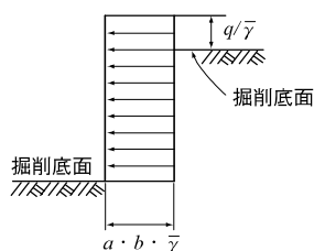
(a) 砂質土地盤土圧
