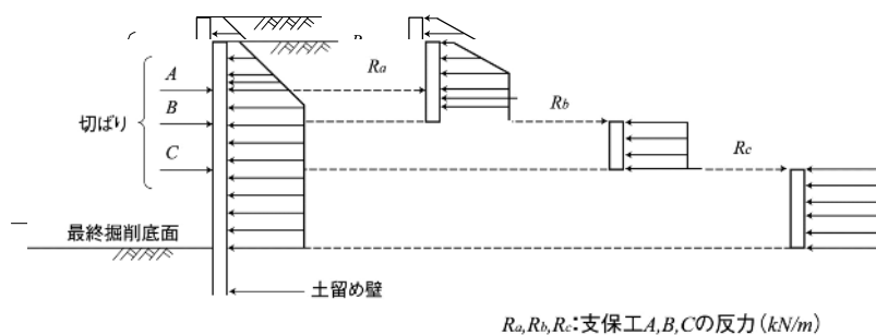
図 1-2-53 腹起しに働く土圧
