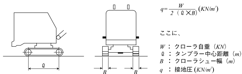
図 1-5-4 クローラクレーンの走行時荷重分布
