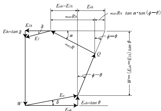
(b) 力の多角形
