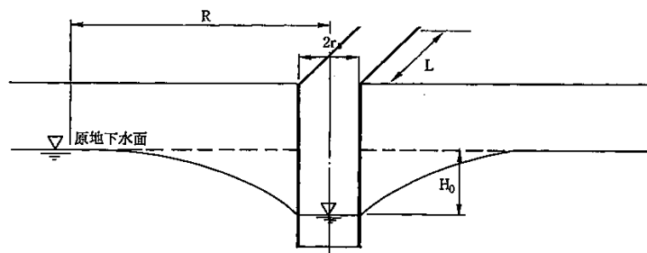
図 1-3-24 不圧帯水層（完全貫入状態）の概念図(2)
