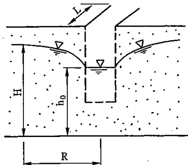
図 1-3-25 不圧帯水層（不完全貫入状態）の概念図
