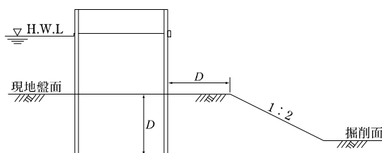
図 1-2-30 望ましい法面形状の例
