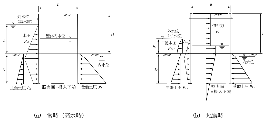
図 1-2-34 滑動の照査モデル 〔二重式仮締切マニュアル 8.2〕
