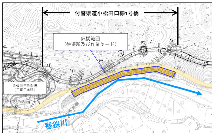
仮橋
