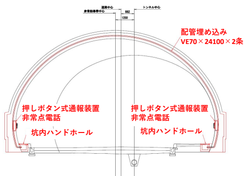
1号トンネル横断図
