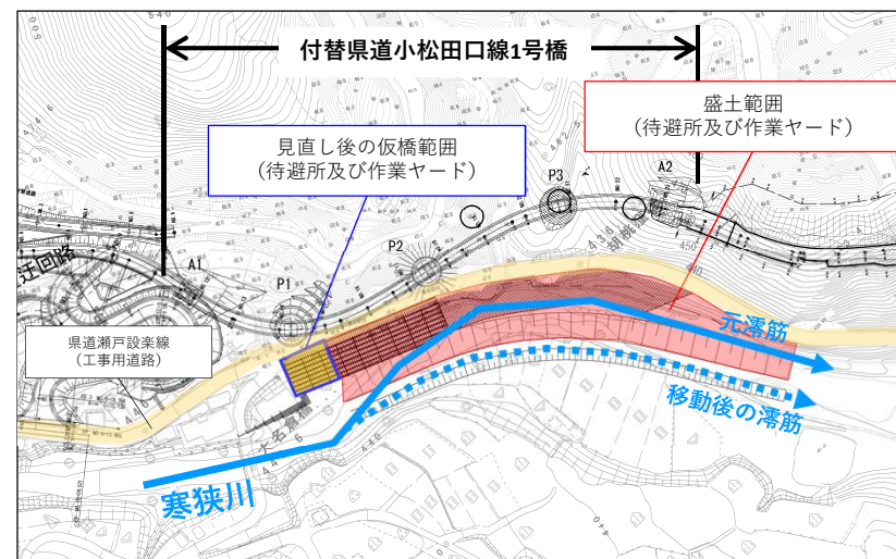
仮橋+盛土
