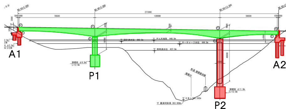
3号橋側面図
