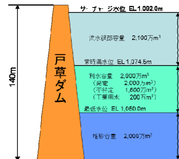
戸草ダム貯水池容量配分図
