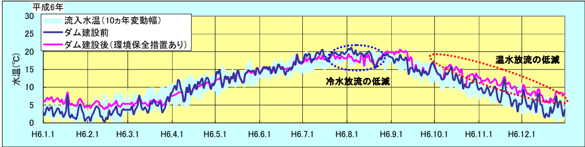
〔環境保全措置がある場合のダム放流水温(平成6年)〕
