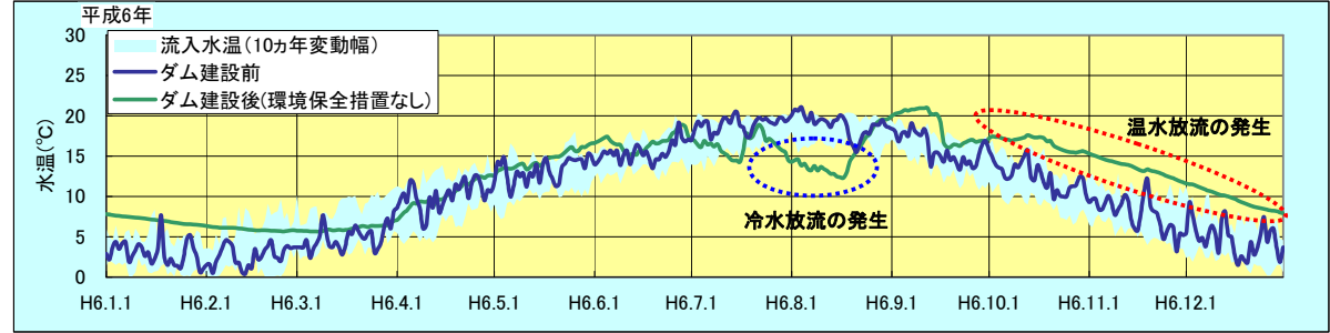
〔環境保全措置がない場合のダム放流水温(平成6年)〕
