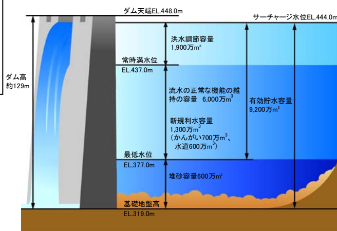
▲設楽ダム容量配分
