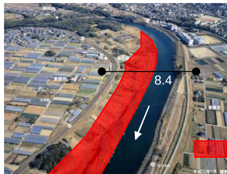
治水対策案の掘削範囲
