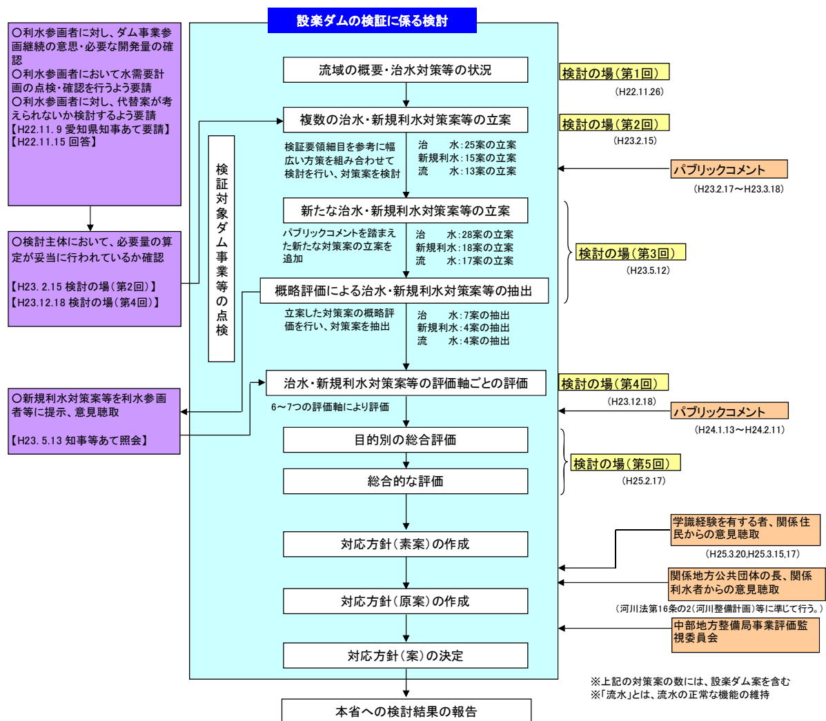
1.1.1 設楽ダム建設事業の検証に係る検討フロー
