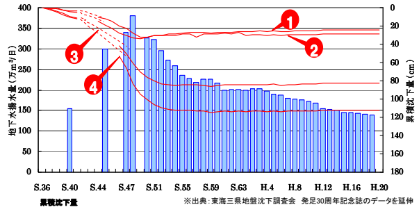
濃尾平野南西部臨海域における一等水準点の地盤沈下と地下水揚水量の経年変動
