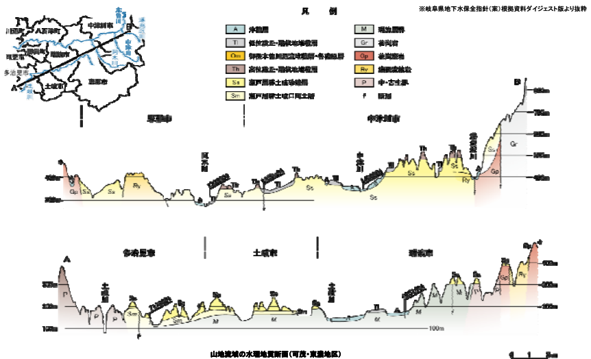
山地流域の水理地質断面(可茂・東濃地区)
