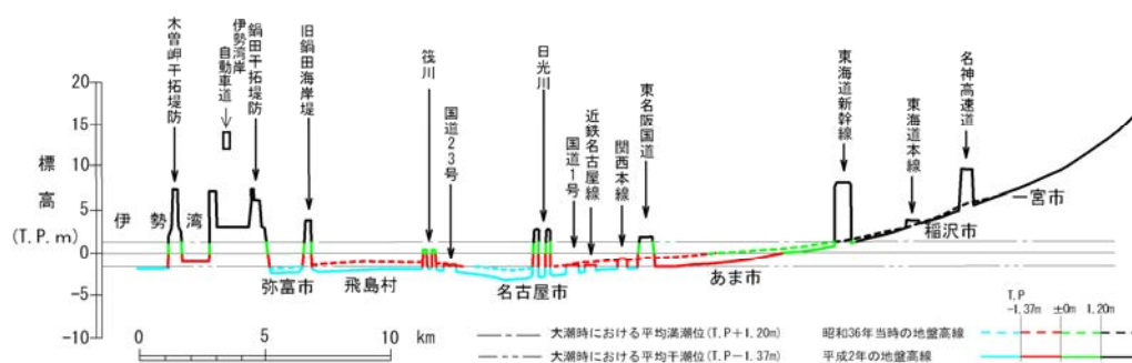
A-A' 断面図
