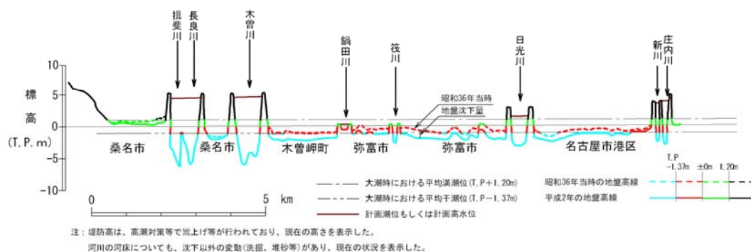
B-B' 断面図
