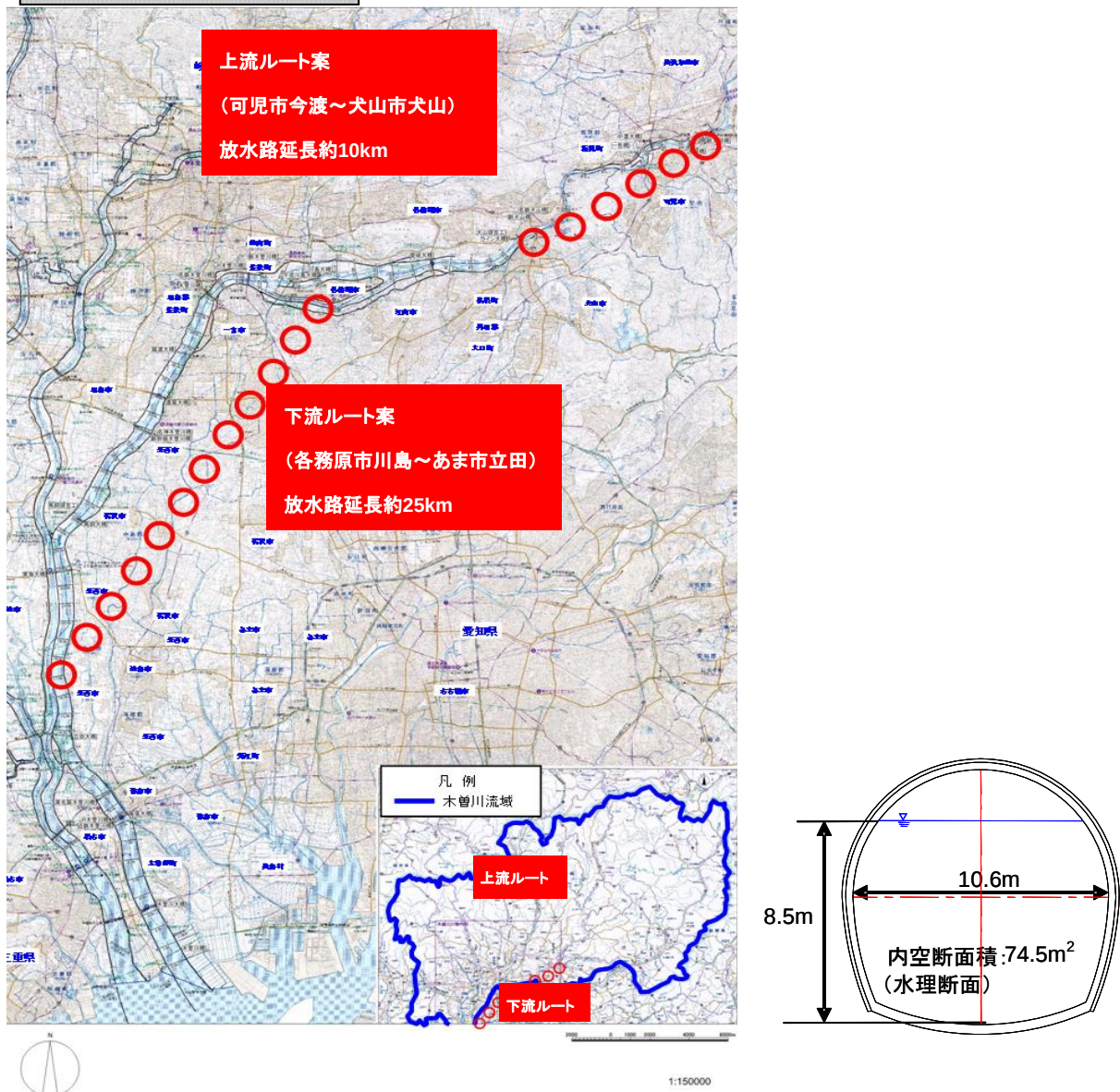
図 4.3.6 放水路（捷水路）のイメージ
