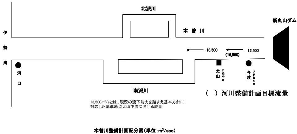
図 4.3.1 木曽川河川整備計画流量図
