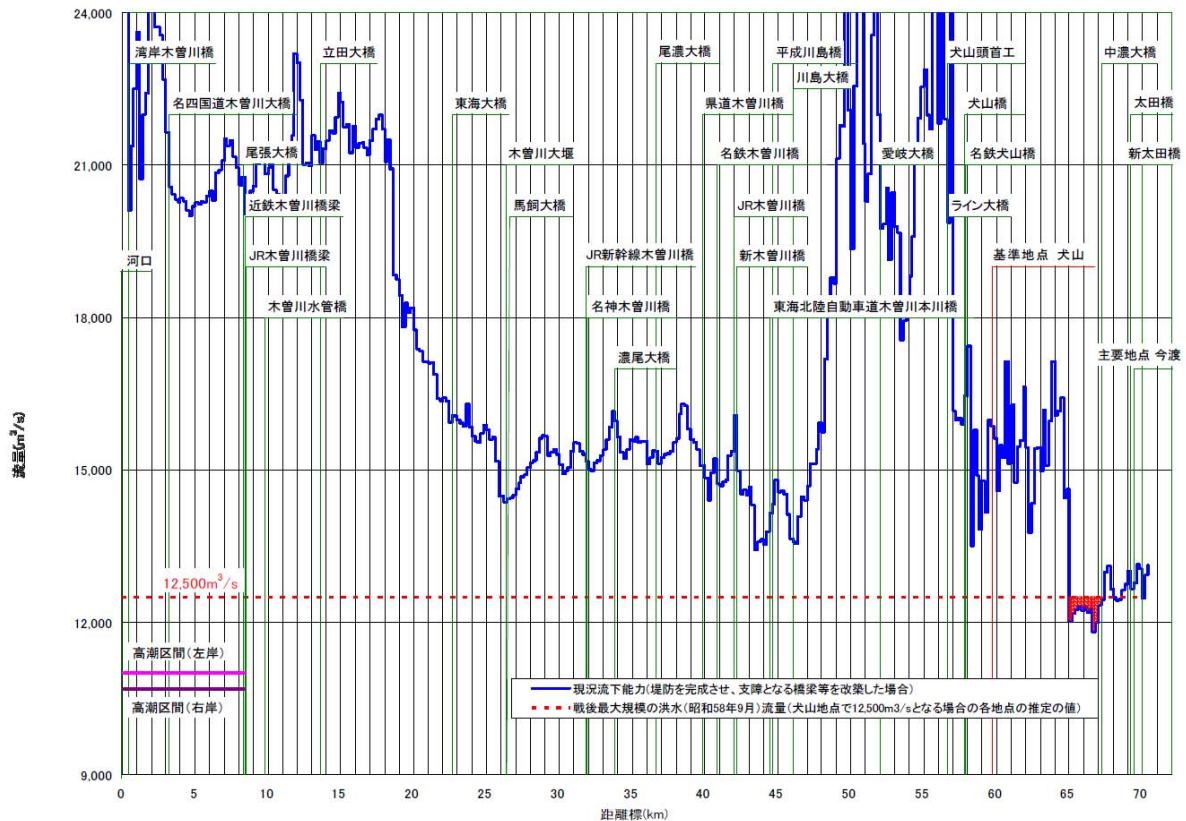
図 4.3.2 流下能力図
