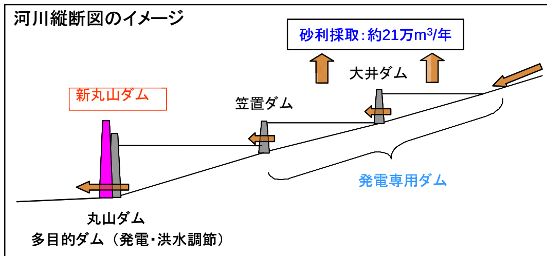
図 4.1.11 丸山・笠置・大井の河川縦断面イメージ
