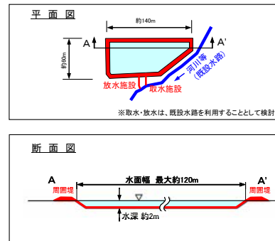
ため池諸元
