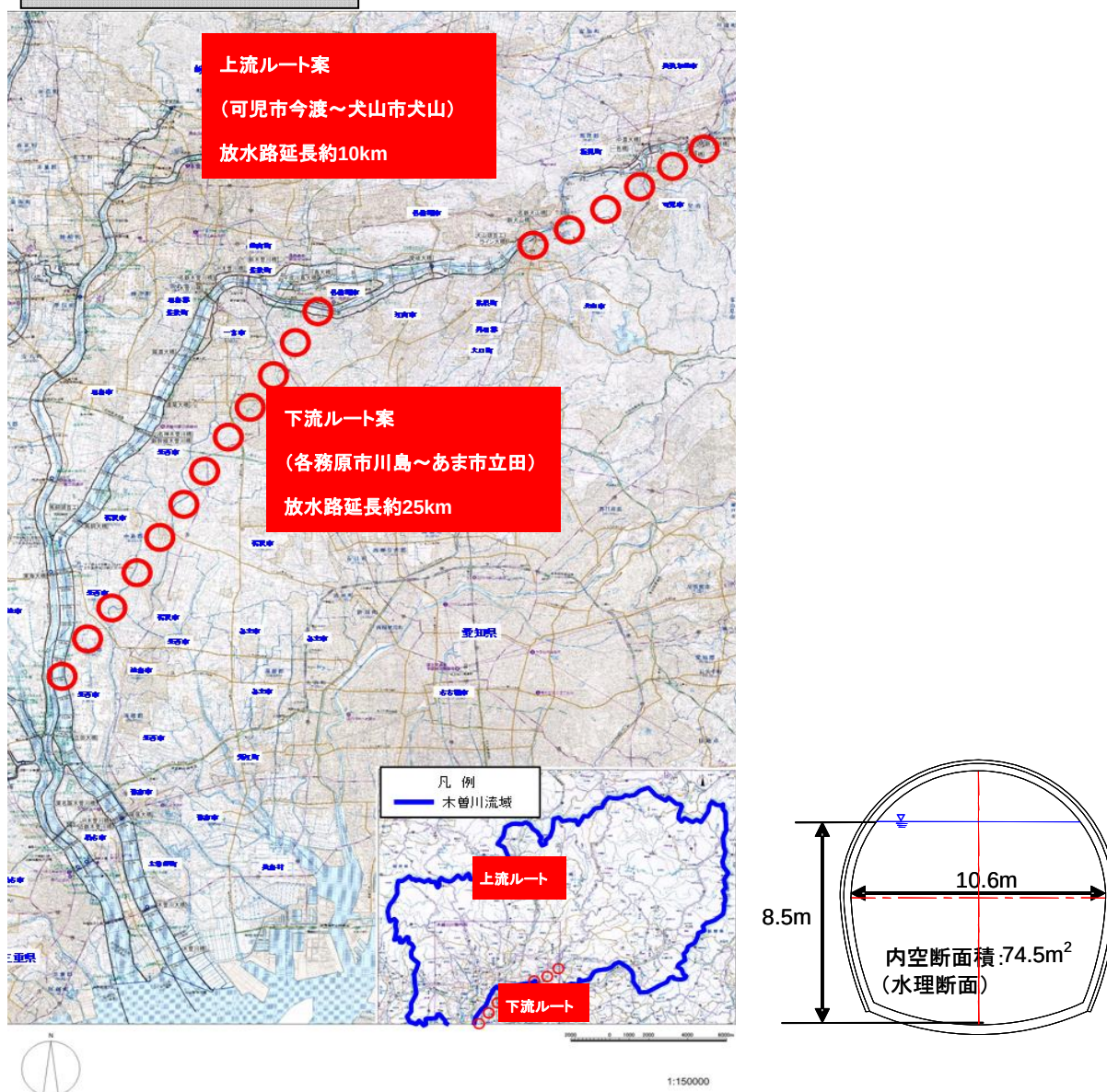
図 4.3.6 放水路（捷水路）のイメージ
