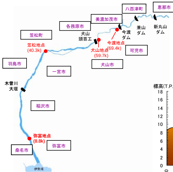
○木曽川位置図
