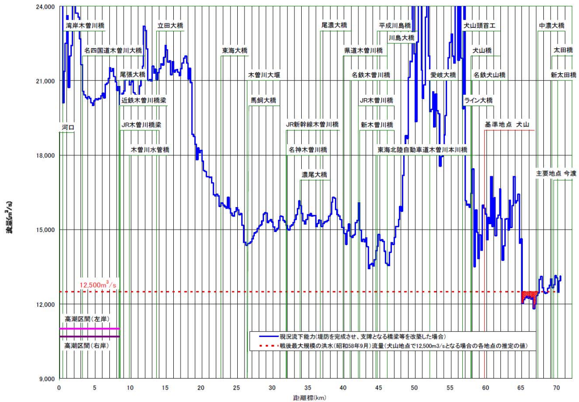
図 4.3.2 流下能力図
