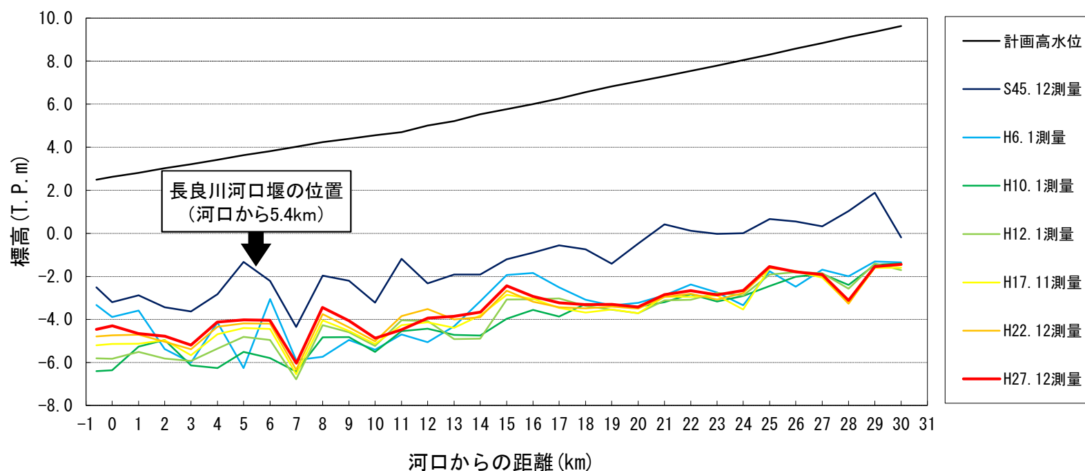
長良川平均河床高(しゅんせつ範囲※内平均)縦断面図
