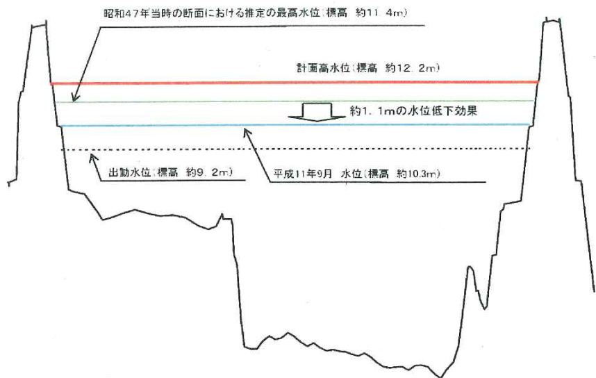
図 1.2.4 水位低下効果図 (H11. 9. 15)
