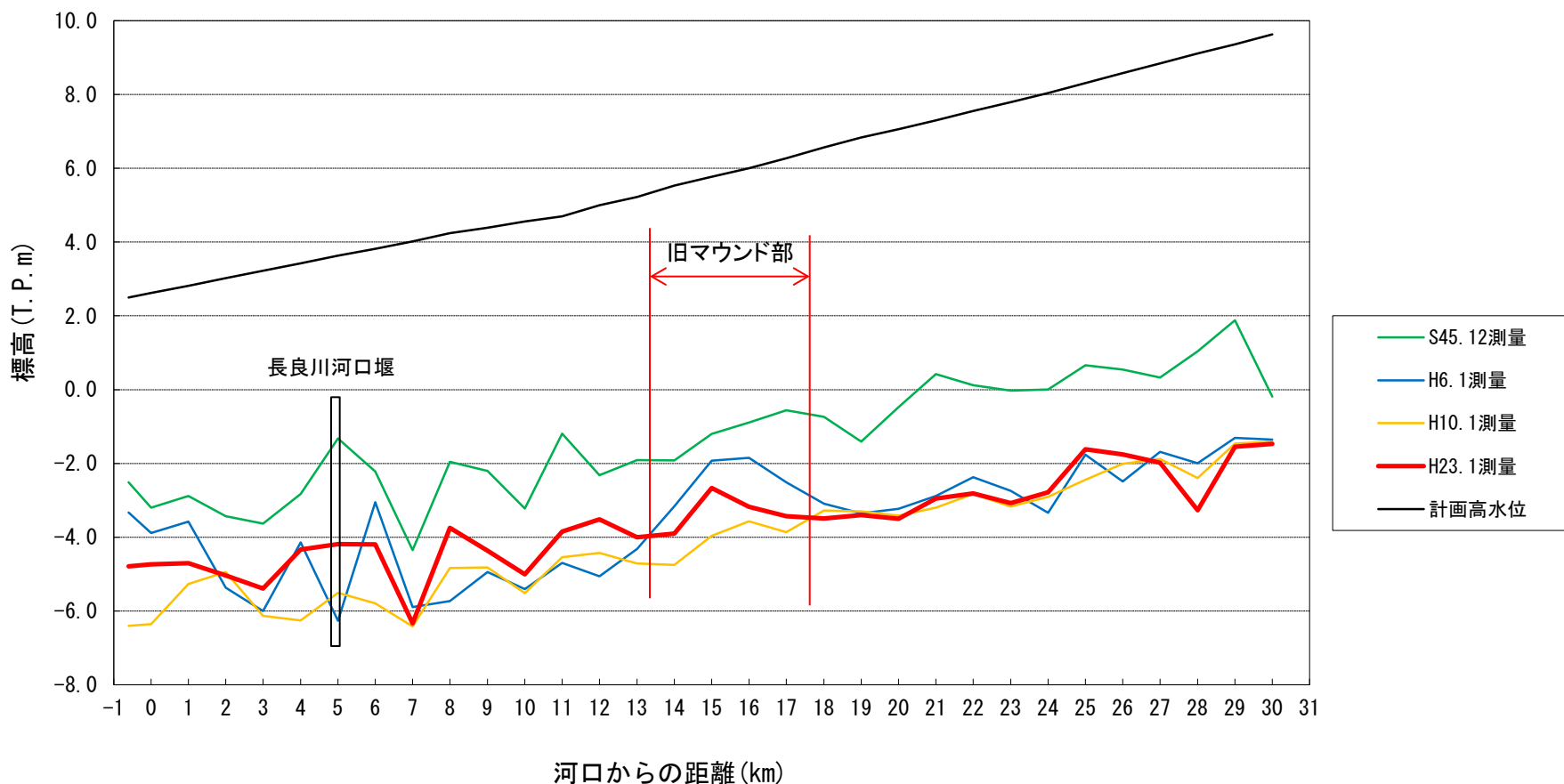
長良川平均河床高(しゅんせつ範囲内平均)縦断図
