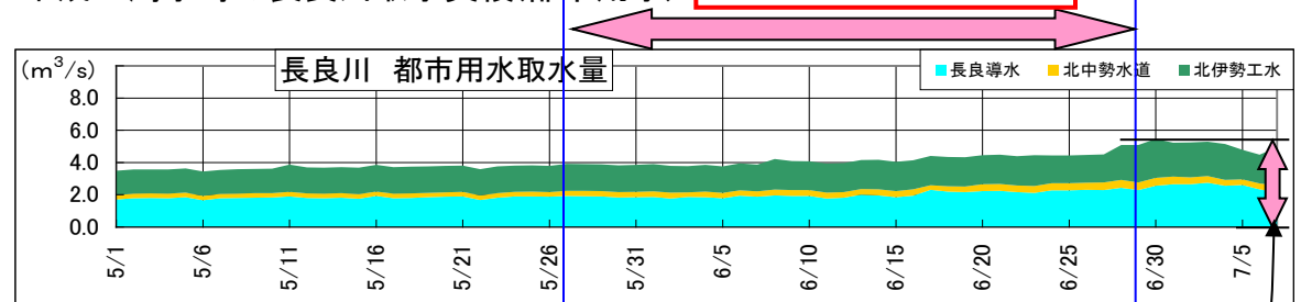
平成17渇水時の長良川取水実績(都市用水)
