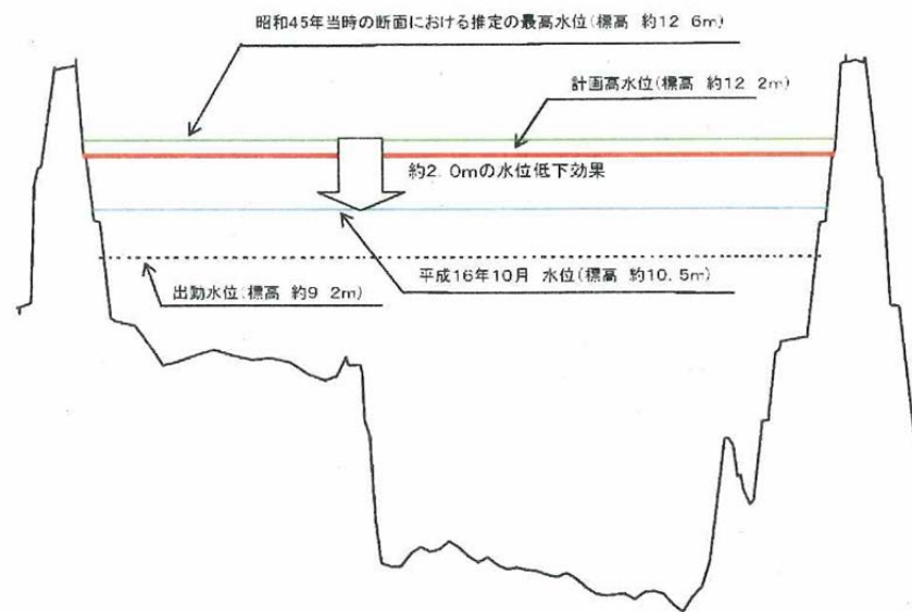
図 1.2.7 水位低下効果図 (H16. 10. 21)
