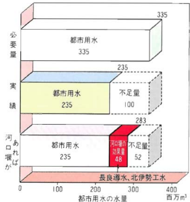
長良川河口堰の完成による効果量(試算)
