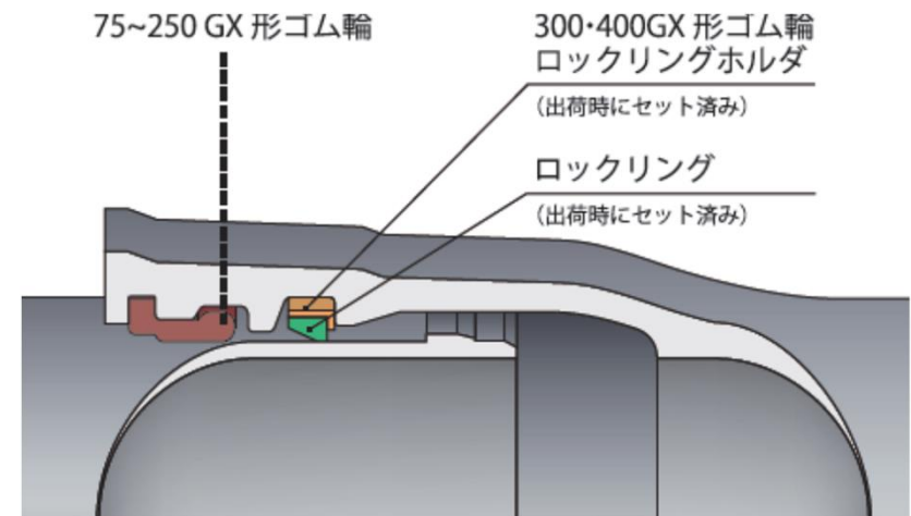
GX形ダクタイル鉄管の構造(直管部) (出典: 日本ダクタイル鉄管協会のパンフレット)
