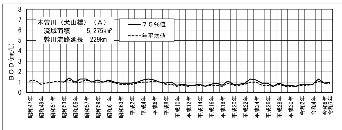
図-4(9.1) 木曽川 犬山橋地点のBOD経年変化
