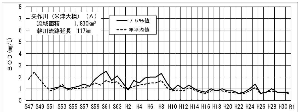
図-4（7） 矢作川米津大橋地点のBOD経年変化
