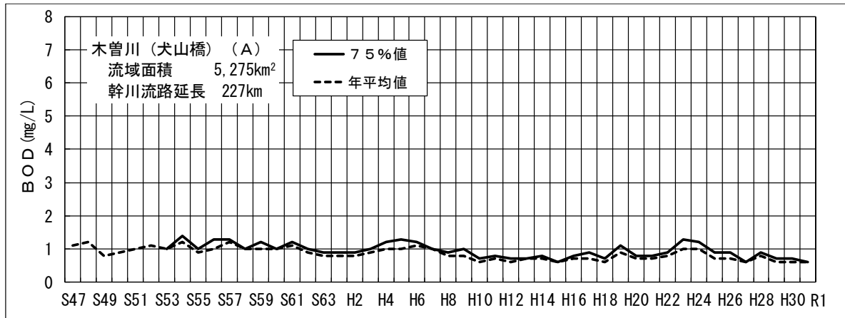
図-4（9-1） 木曾川犬山橋地点のBOD経年変化
