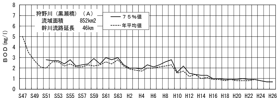
図－４（１） 狩野川黒瀬橋地点のBOD経年変化
