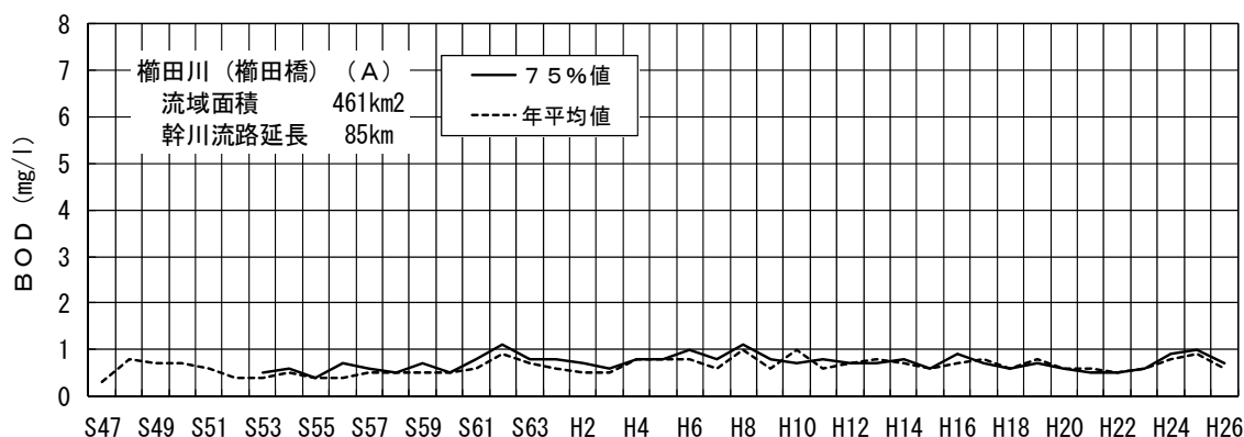
図－4（1 2） 櫛田川櫛田橋地点のBOD経年変化
