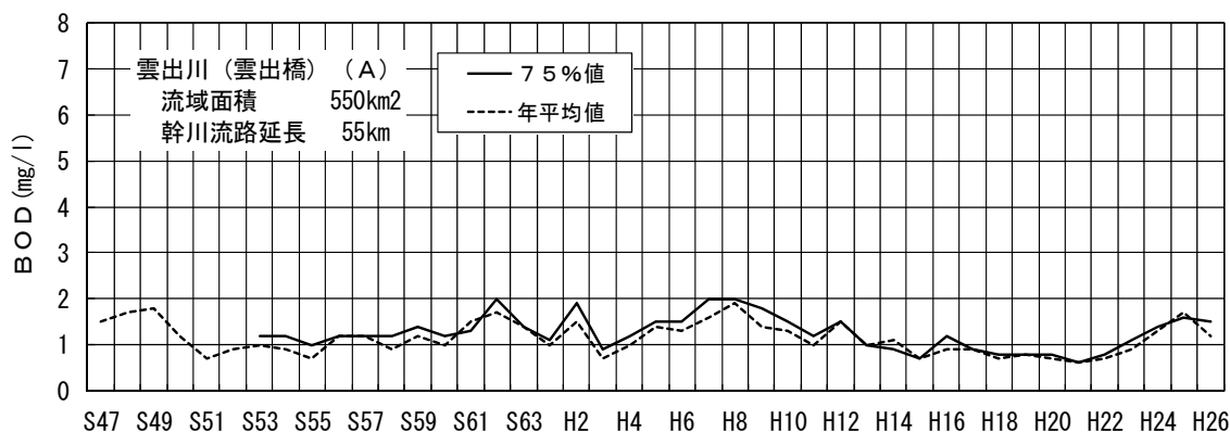
図－4（11） 雲出川雲出橋地点のBOD経年変化
