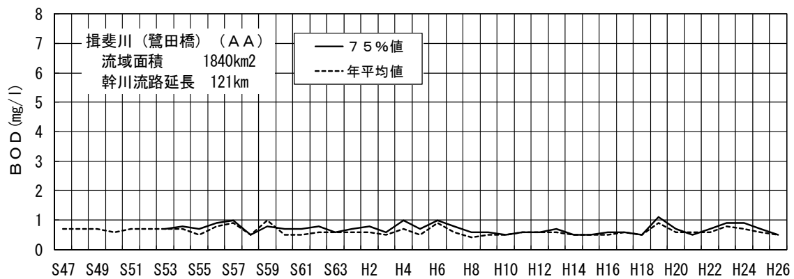
図－４（９－５） 揖斐川鷺田橋地点のＢＯＤ経年変化
