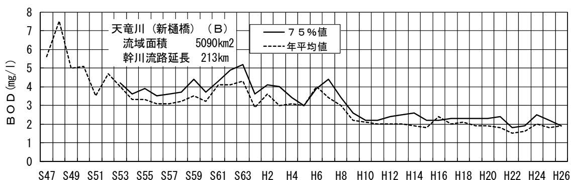
図－4（5－1） 天竜川上流部（新樋橋地点）のBOD経年変化
