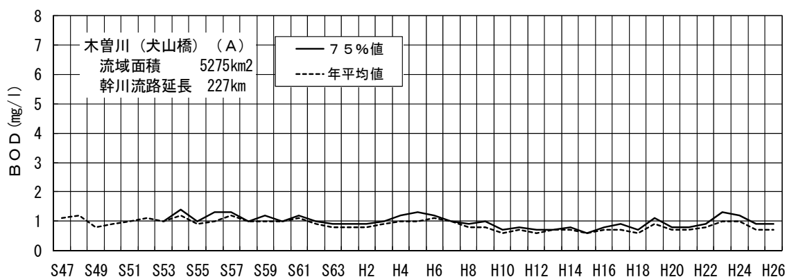
図－4（9－1） 木曽川犬山橋地点のBOD経年変化
