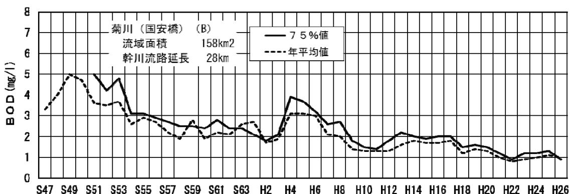
図－4（4） 菊川国安橋地点BOD経年変化
