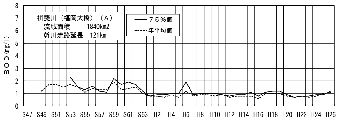
図－４（９－６） 揖斐川福岡大橋地点のＢＯＤ経年変化
