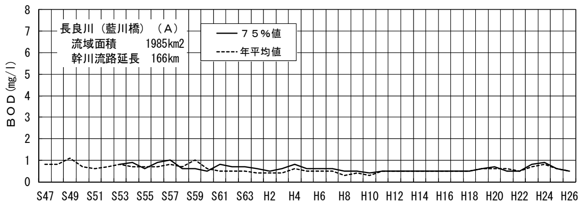
図－４（９－３） 長良川藍川橋地点のBOD経年変化
