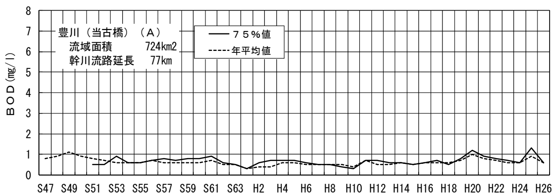
図－4（6） 豊川当古橋地点のBOD経年変化
