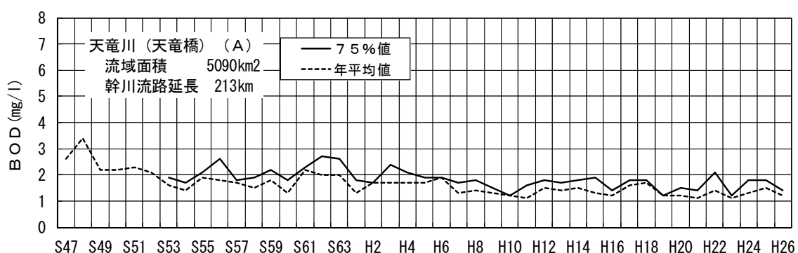
図－4（5－2） 天竜川中流部（天竜橋地点）のBOD経年変化
