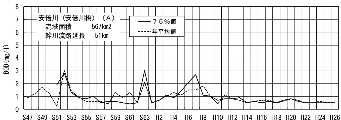
図－４（２） 安倍川安倍川橋地点のBOD経年変化
