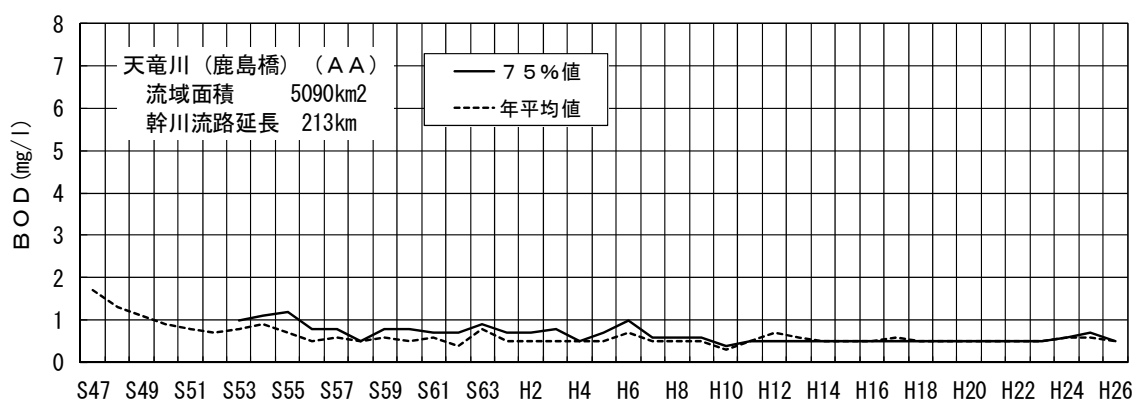
図－4（5－3） 天竜川下流部（鹿島橋地点）のBOD経年変化
