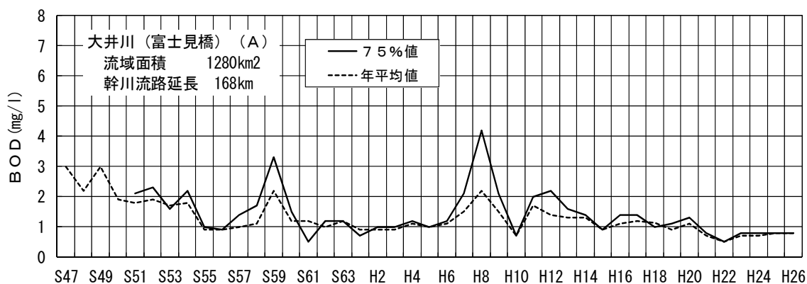
図－4（3） 大井川富士見橋地点のBOD経年変化
