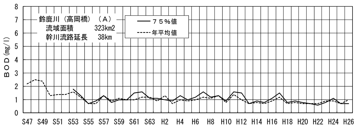
図－4（10） 鈴鹿川高岡橋地点のBOD経年変化
