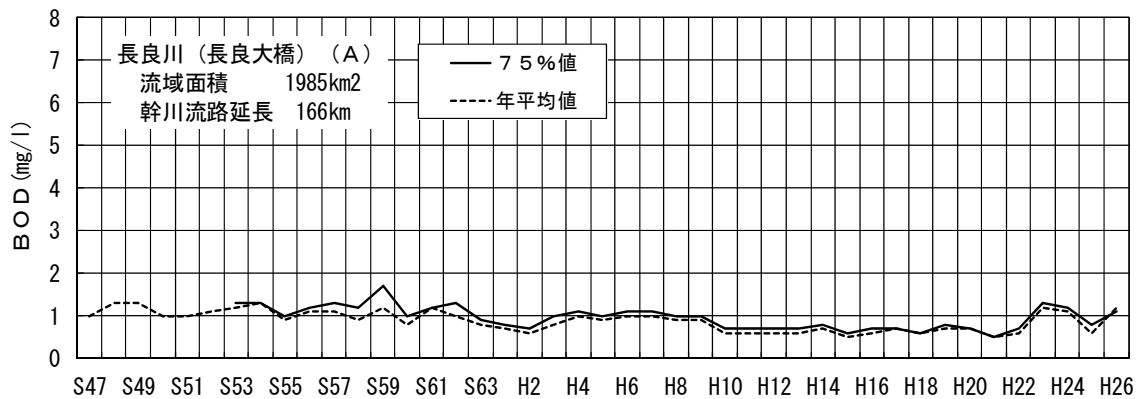
図－４（９－４） 長良川長良大橋地点のBOD経年変化
