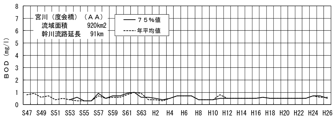
図－4（1 3） 宮川度会橋地点のBOD経年変化
