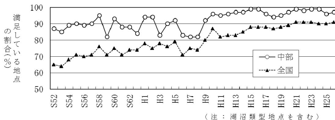
図－2 一級河川における環境基準を満足している地点割合の経年変化
