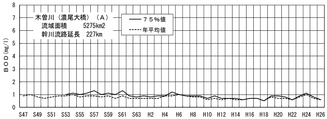
図－４（９－２） 木曽川濃尾大橋地点のBOD経年変化
