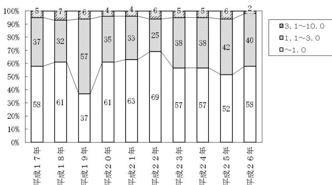
図－３ ＢＯＤ７５％値ランク別経年割合
