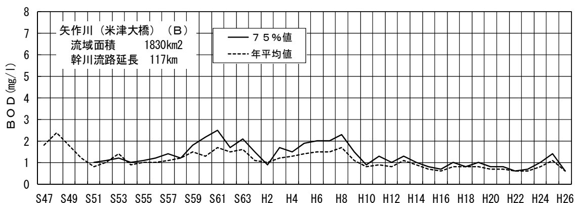
図－4（7） 矢作川米津大橋地点のBOD経年変化
