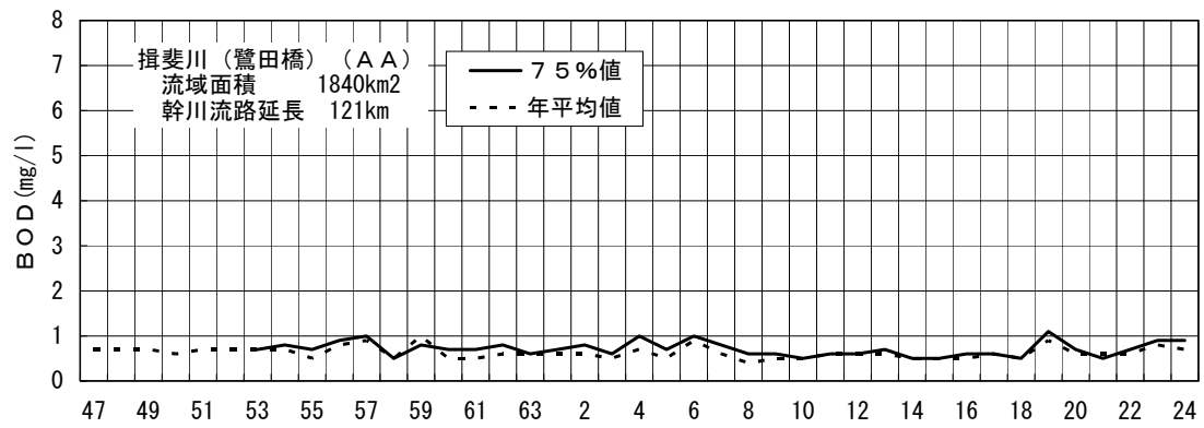
図-4 (9-5) 揖斐川鷺田橋地点のBOD経年変化
