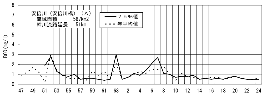
図－4（2） 安倍川安倍川橋地点のBOD経年変化
