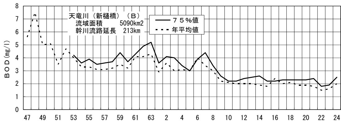
図-4(5-1) 天竜川上流部(新樋橋地点)のBOD経年変化
