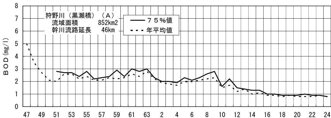
図－4（1） 狩野川黒瀬橋地点のBOD経年変化
