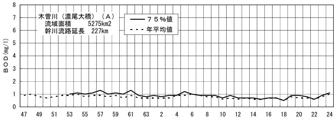
図-4（9-2） 木曾川濃尾大橋地点のBOD経年変化
