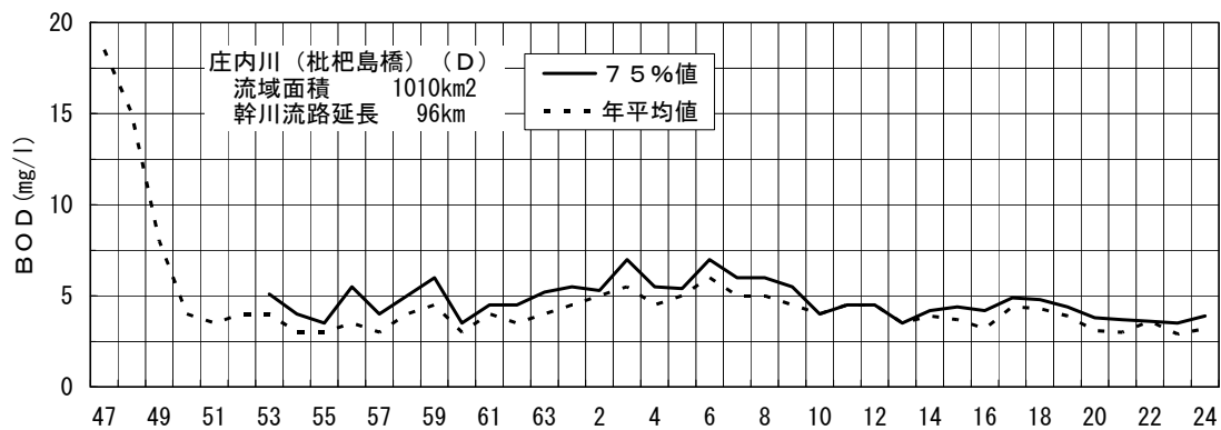
図-4（8） 庄内川枇杷島橋地点のBOD経年変化
