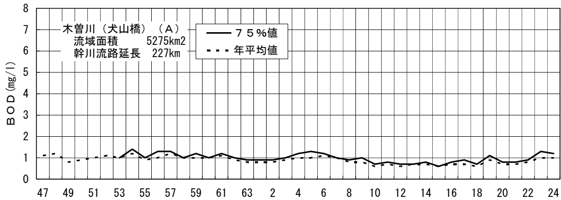
図-4（9-1） 木曾川犬山橋地点のBOD経年変化
