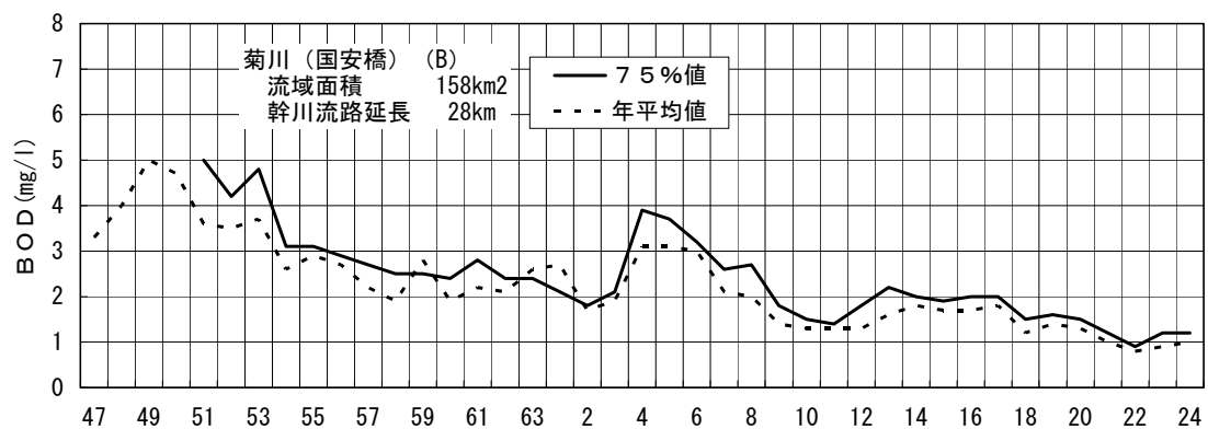
図-4（4） 菊川国安橋地点BOD経年変化
