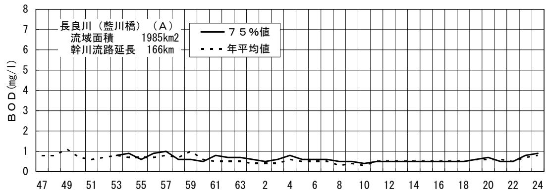
図-4（9-3） 長良川藍川橋地点のBOD経年変化
