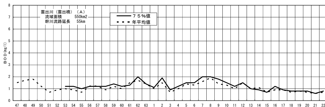
図-5（11） 雲出川雲出橋地点のBOD経年変化
