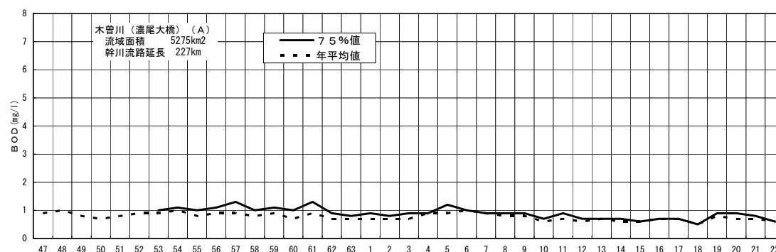
図-5（9-2） 木曾川濃尾大橋地点のBOD経年変化
