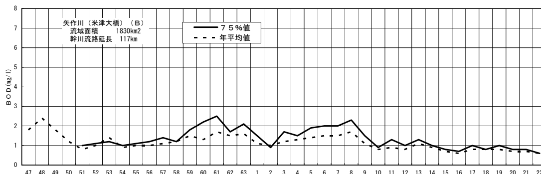
図－5（7） 矢作川米津大橋地点のBOD経年変化
