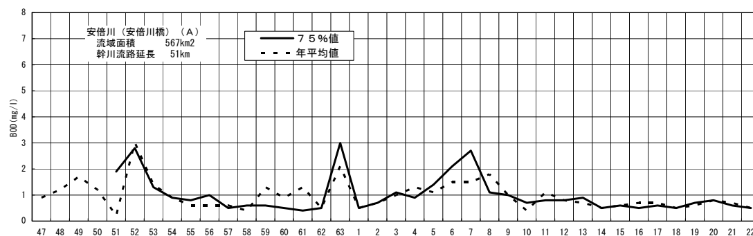
図－5（2） 安倍川安倍川橋地点のBOD経年変化
