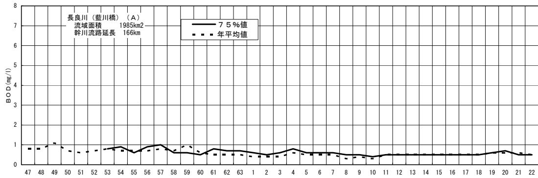
図-5 (9-3) 長良川藍川橋地点のBOD経年変化
