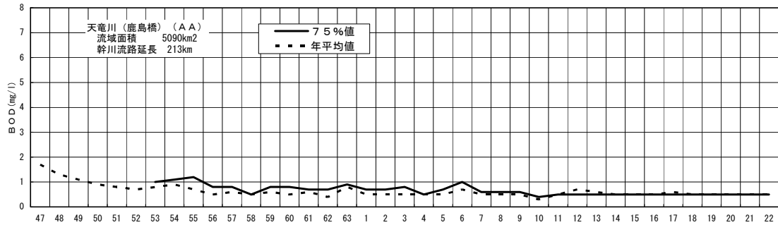
図-5 (5-3) 天竜川下流部(鹿島橋地点)のBOD経年変化
