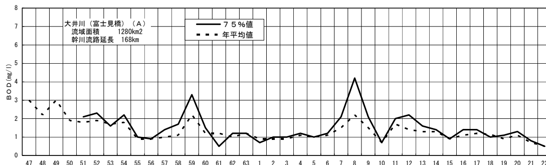
図－5（3） 大井川富士見橋地点のBOD経年変化
