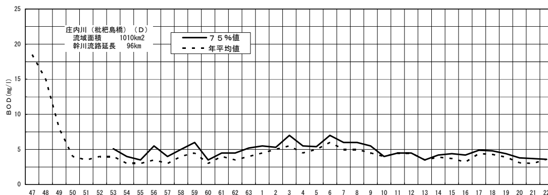
図－5（8） 庄内川枇杷島橋地点のBOD経年変化
