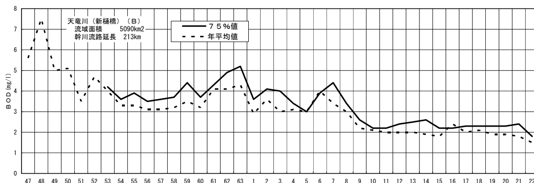
図-5(5-1) 天竜川上流部（新樋橋地点）のBOD経年変化
