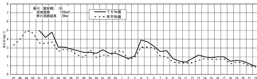
図－5（4） 菊川国安橋地点BOD経年変化
