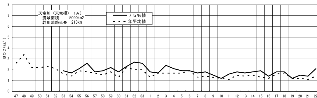
図-5(5-2) 天竜川中流部（天竜橋地点）のBOD経年変化
