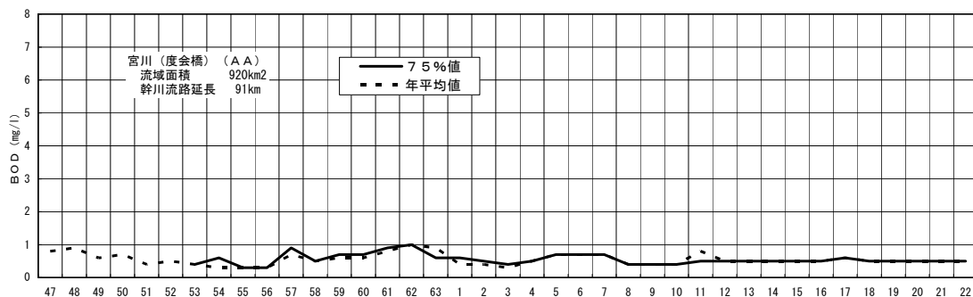
図－5（13） 宮川度会橋地点のBOD経年変化
