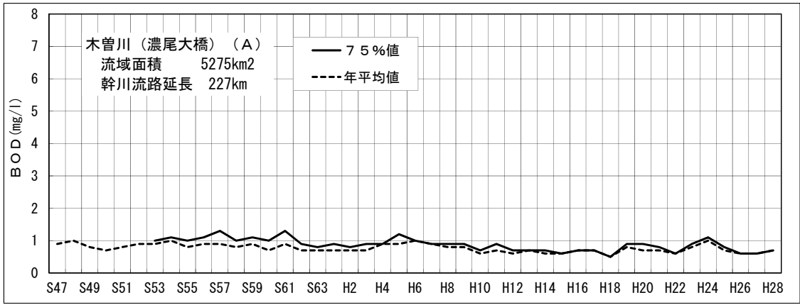
図-4（9-2） 木曽川濃尾大橋地点のBOD経年変化
