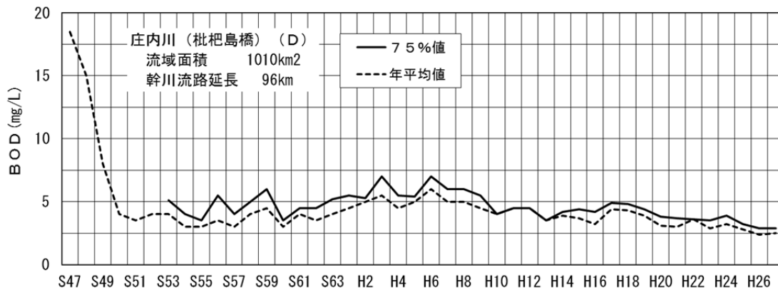
図-4（8） 庄内川枇杷島橋地点のBOD経年変化
