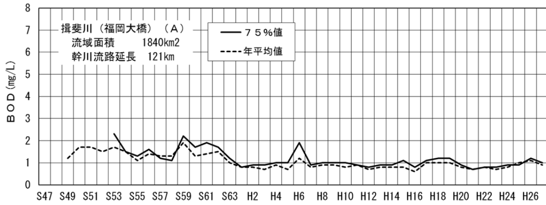
図-4 (9-6) 揖斐川福岡大橋地点のBOD経年変化
