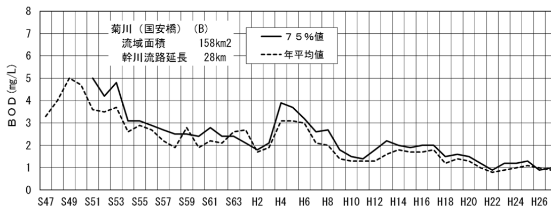
図－4（4） 菊川国安橋地点BOD経年変化
