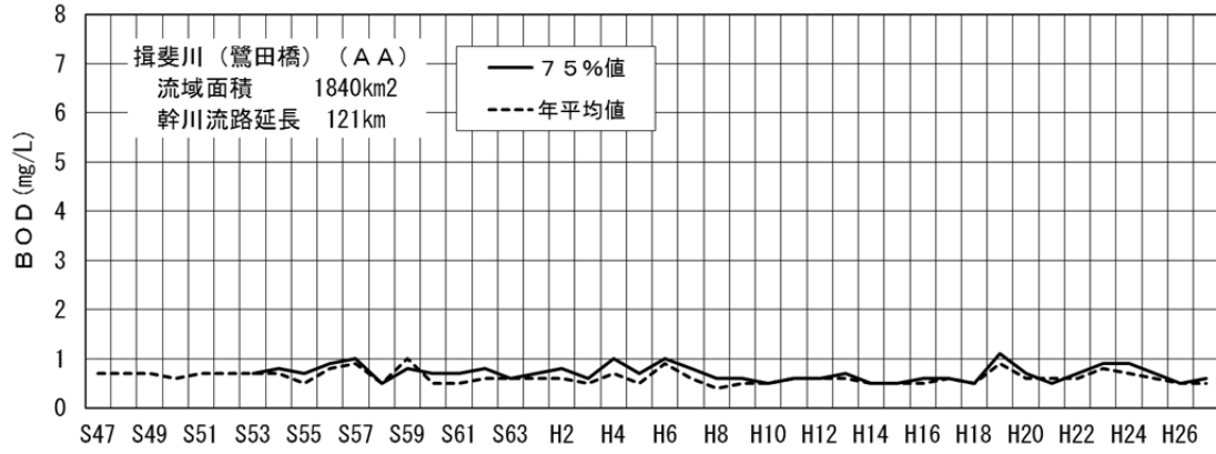
図-4 (9-5) 揖斐川鷺田橋地点のBOD経年変化
