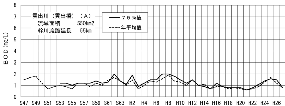
図-4（11） 雲出川雲出橋地点のBOD経年変化
