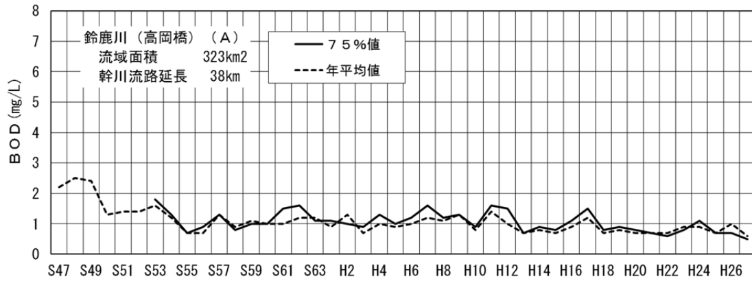
図-4（10） 鈴鹿川高岡橋地点のBOD経年変化
