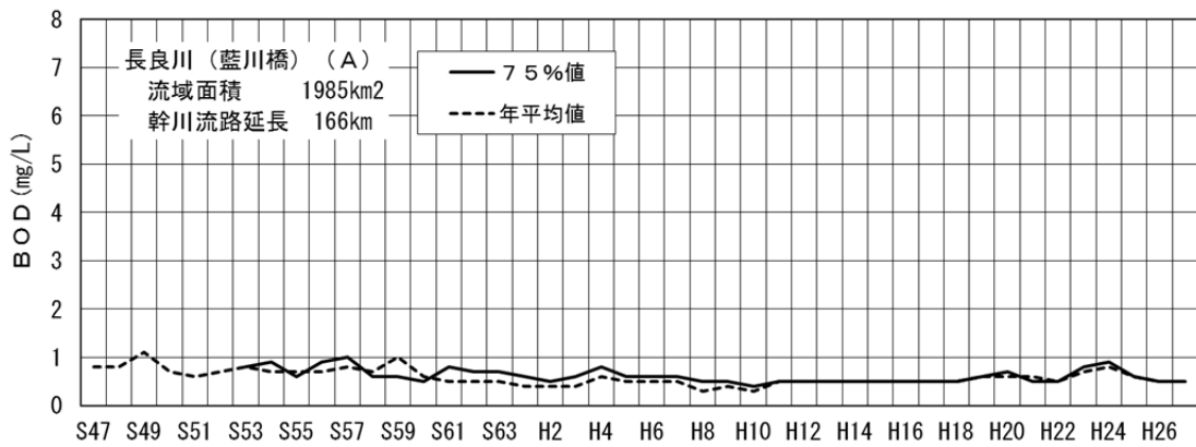
図-4 (9-3) 長良川藍川橋地点のBOD経年変化
