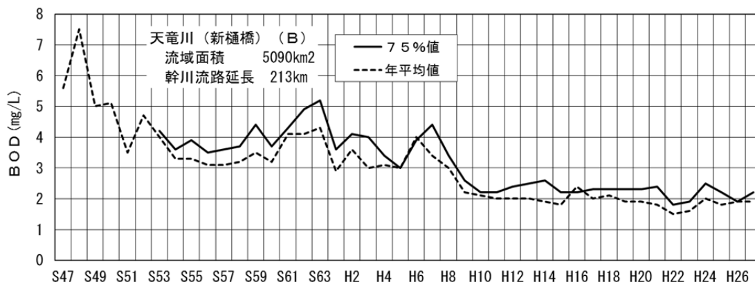
図-4(5-1) 天竜川上流部(新樋橋地点)のBOD経年変化
