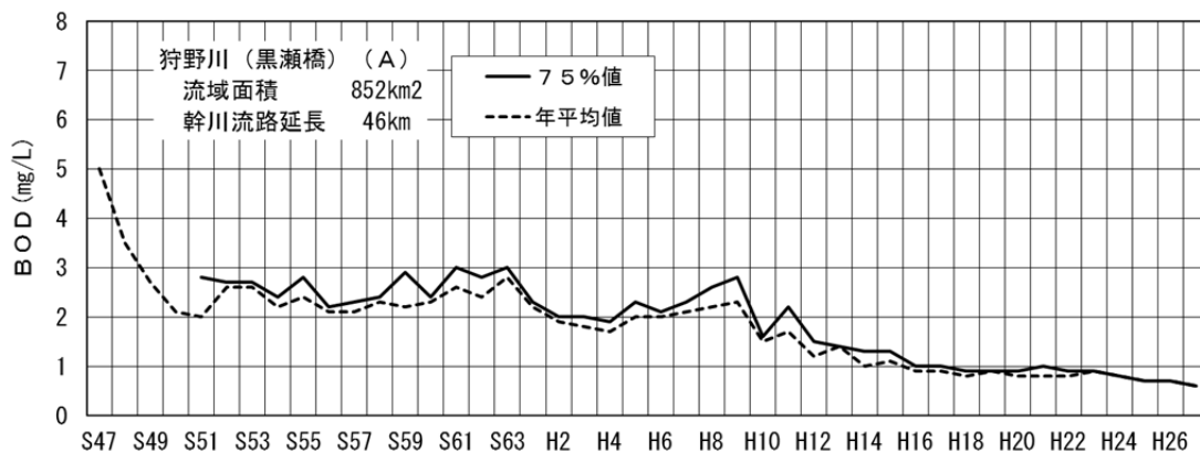
図－4（1） 狩野川黒瀬橋地点のBOD経年変化
