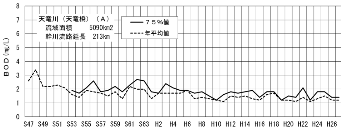
図-4(5-2) 天竜川中流部(天竜橋地点)のBOD経年変化
