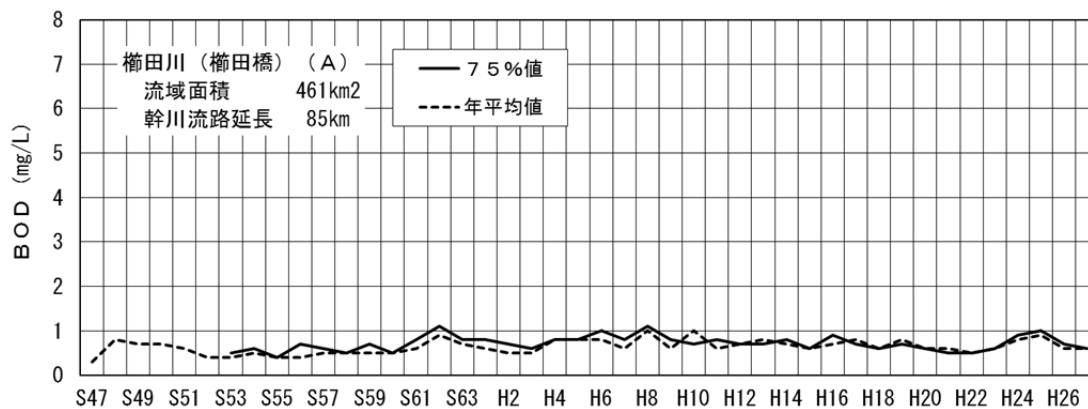
図-4（12） 櫛田川櫛田橋地点のBOD経年変化
