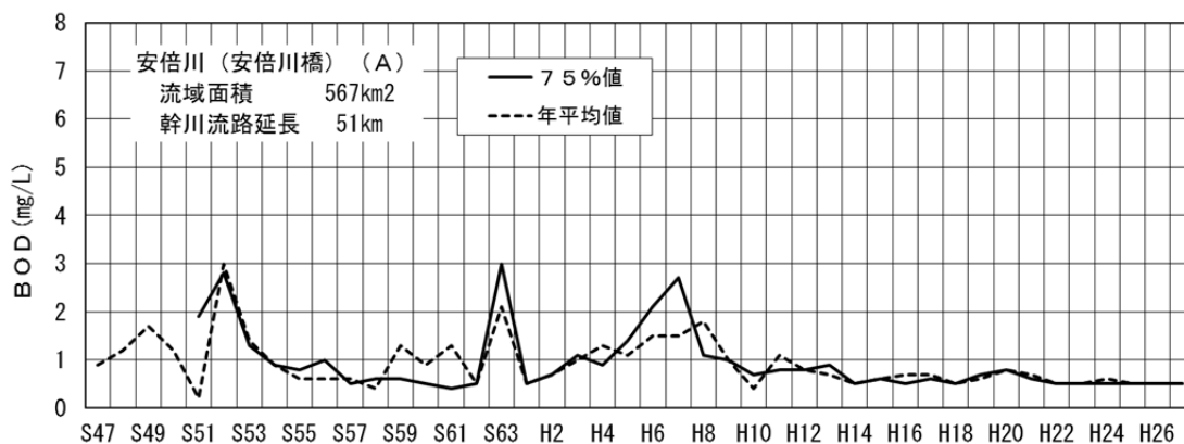
図－4（2） 安倍川安倍川橋地点のBOD経年変化
