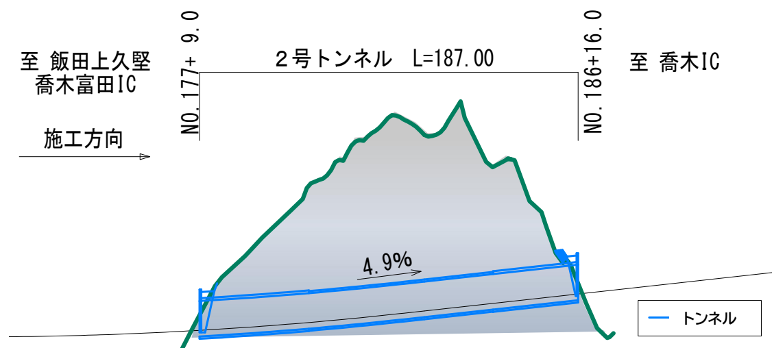
トンネル一般図
