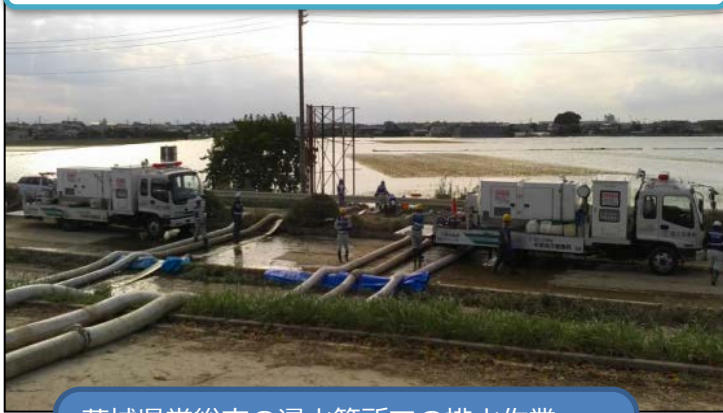
茨城県常総市の浸水箇所での排水作業 (天竜川上流の照明車・排水ポンプ車 H27.9/10~18)
