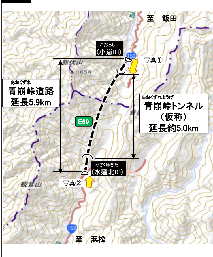
全体図
