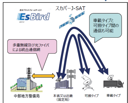
【衛星小型画像伝送装置 (Ku-Sat) で通信訓練】
