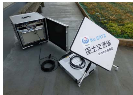
Ku-SAT(可搬型)
