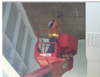
高所作業車による点検事例 （講習会では大型のものを使用します）
