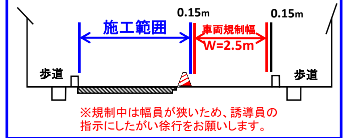
【施工断面図】
