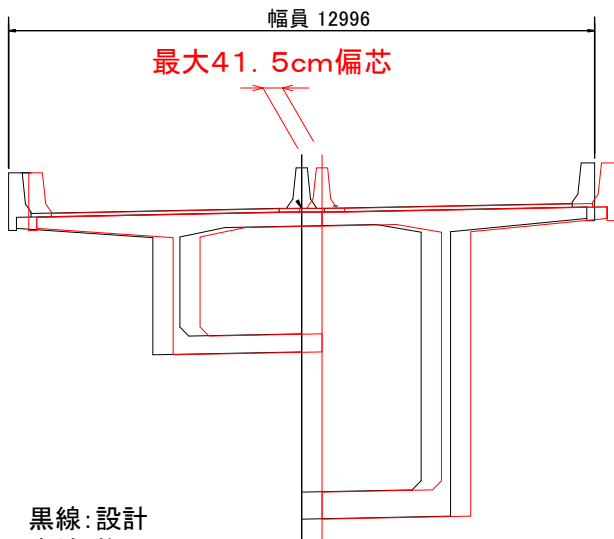
橋梁断面図
