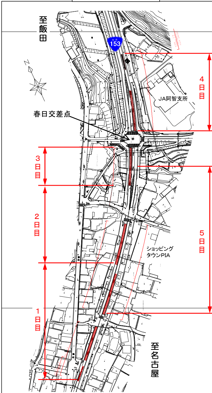
工事施工箇所図
