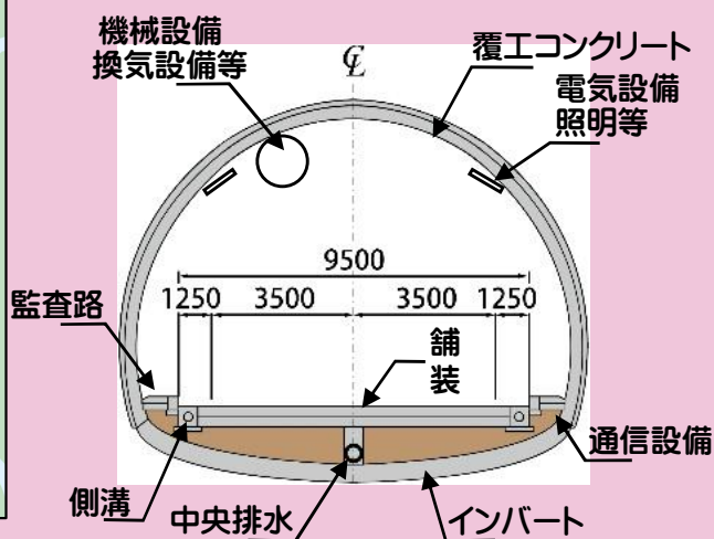
トンネル断面図
