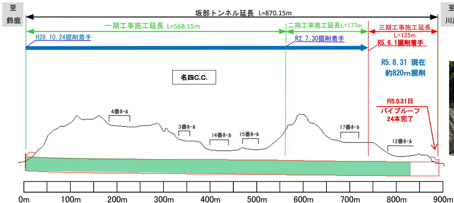
施工状況（令和5年8月度）
