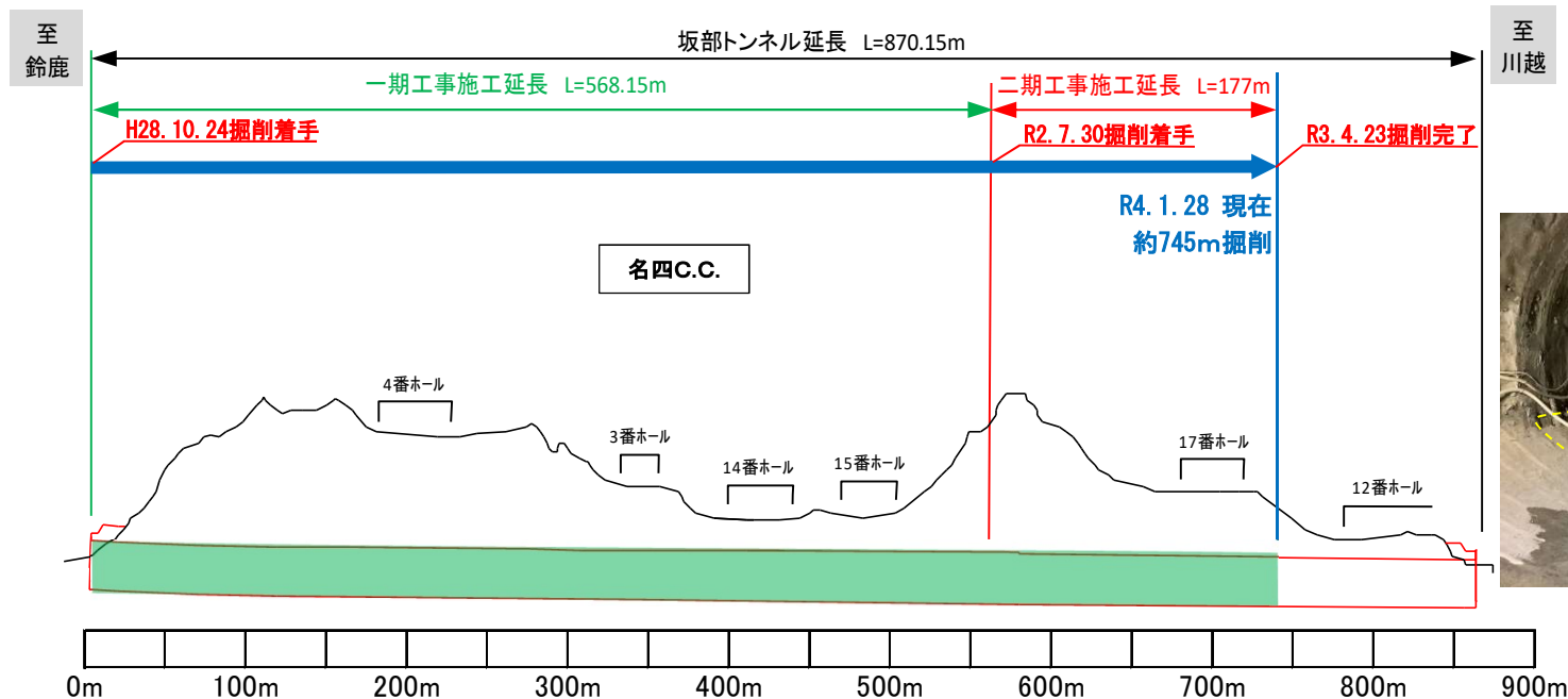
施工状況（令和4年1月度）
