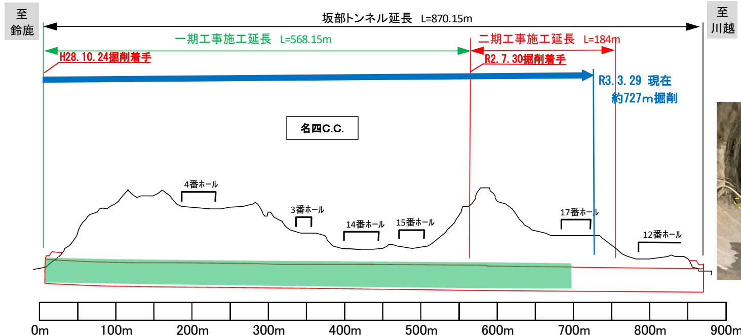
施工状況（令和3年3月度）
